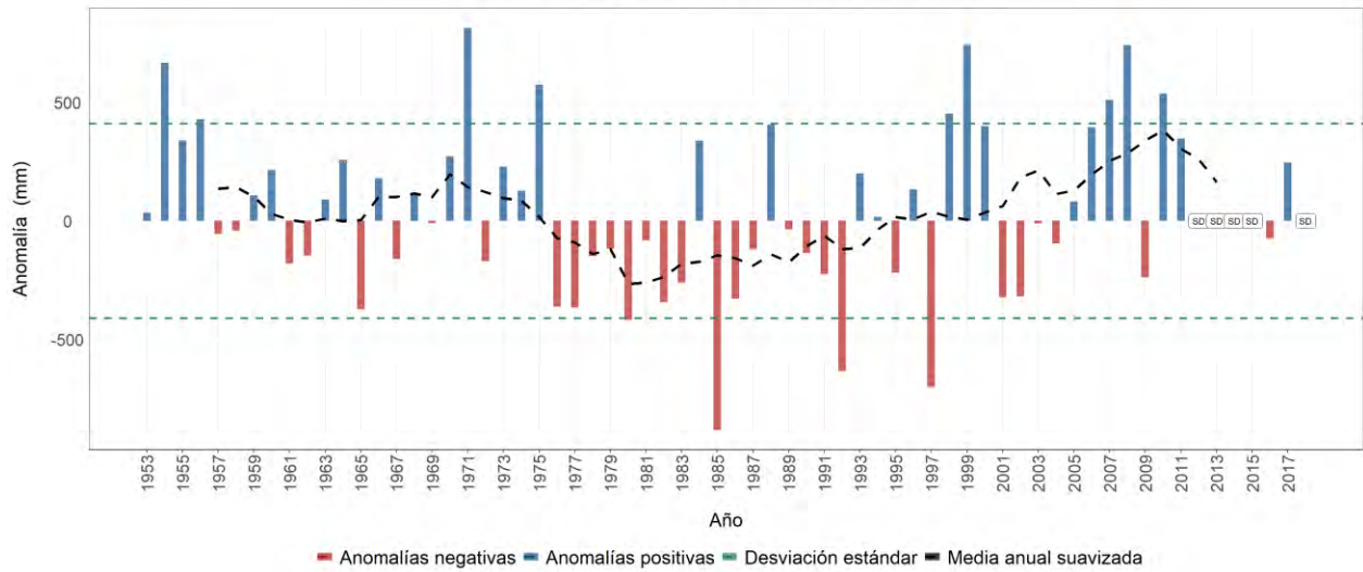
Estación meteorológica 2619501 - MIGUEL VALENCIA, Jardín, Antioquia Evolución anual de la anomalía de precipitación Promedio del periodo base (1981-2010): 2116 mm
