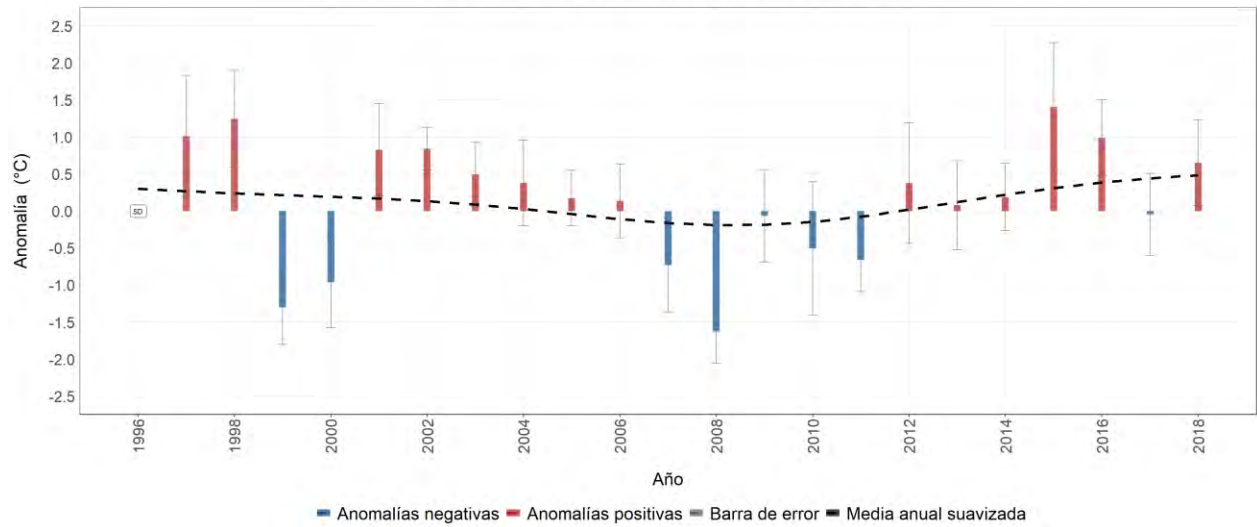
Estación meteorológica 5203503 - EL SAUCE, La Unión, Nariño Evolución anual de la anomalía de temperatura máxima media Promedio del período base (1981-2010): 25.7 °C
