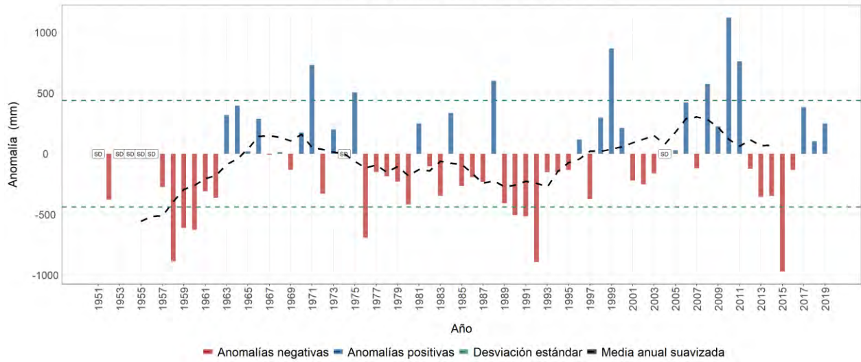
Estación meteorológica 2612006 - ALMACAFÉ VIVERO, Quimbaya, Quindío Evolución anual de la anomalía de precipitación Promedio del período base (1981-2010): 2221 mm
