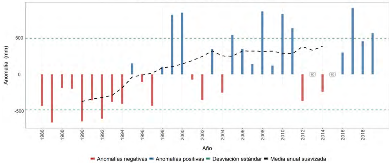
Estación meteorológica 2613052 - LA ARGENTINA, Palestina, Caldas Evolución anual de la anomalía de precipitación Promedio del periodo base (1981-2010): 2590 mm
