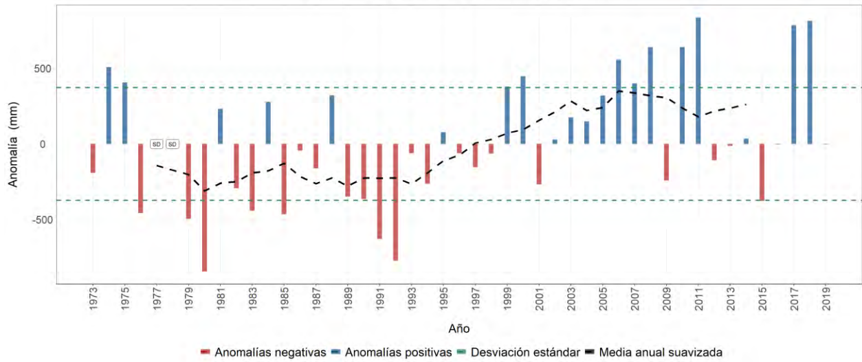
Estación meteorológica 2612044 - LA ARGENTINA, La Tebaida, Quindío Evolución anual de la anomalía de precipitación Promedio del periodo base (1981-2010): 2069 mm
