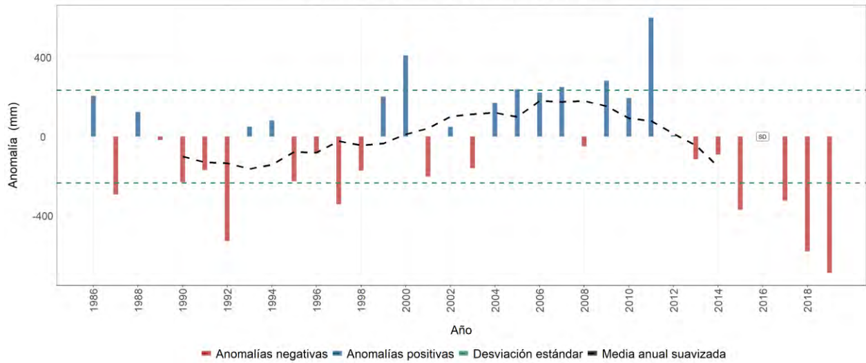
Estación meteorológica 2103010 - CONCENTRACIÓN DESARROLLO, Timaná, Huila Evolución anual de la anomalía de precipitación Promedio del periodo base (1981-2010): 1244 mm
