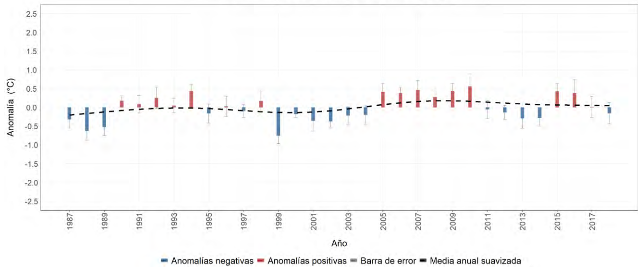
Estación meteorológica 2612523 - EL AGRADO, Montenegro, Quindío Evolución anual de la anomalía de temperatura mínima media Promedio del periodo base (1981-2010): 16.9 °C
