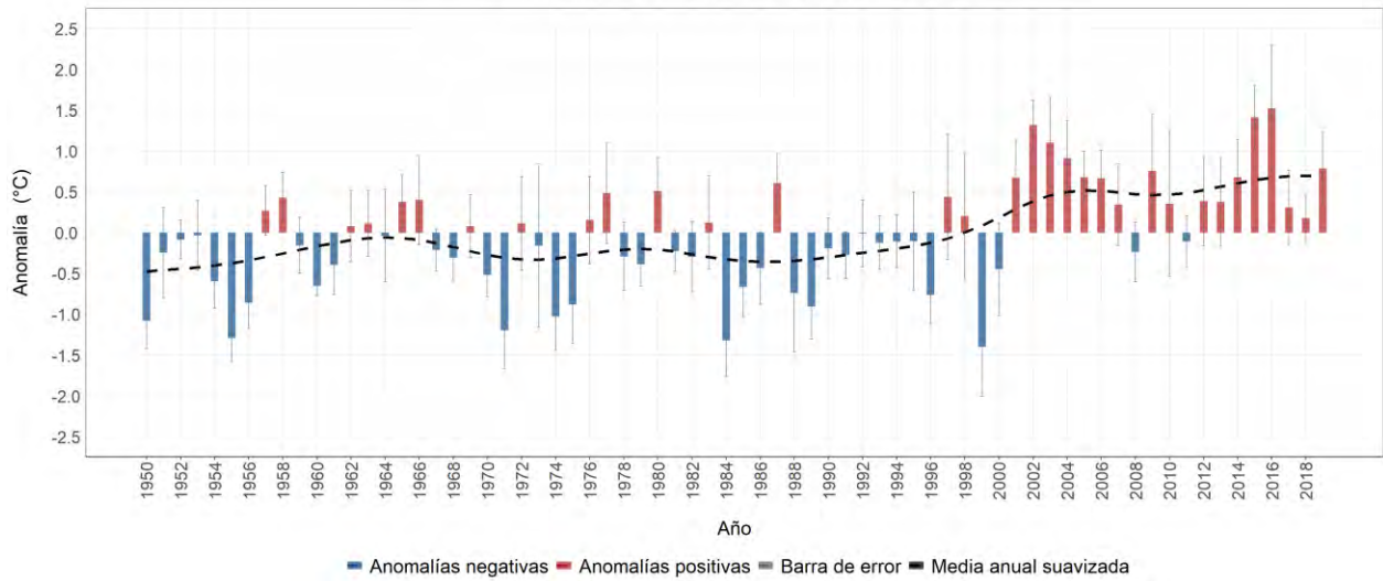
Estación meteorológica 2615502 - CENICAFÉ, Chinchiná, Caldas Evolución anual de la anomalía de temperatura máxima media Promedio del período base (1981-2010): 27.7 °C
