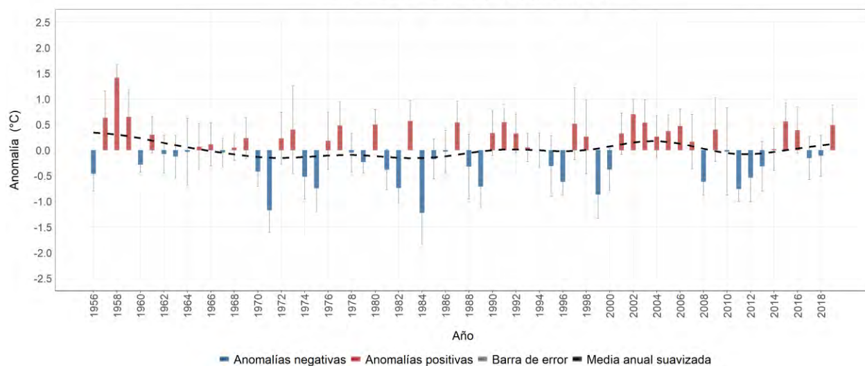
Estación meteorológica 2613505 - NARANJAL, Chinchiná, Caldas Evolución anual de la anomalía de temperatura máxima media Promedio del período base (1981-2010): 26.8 °C
