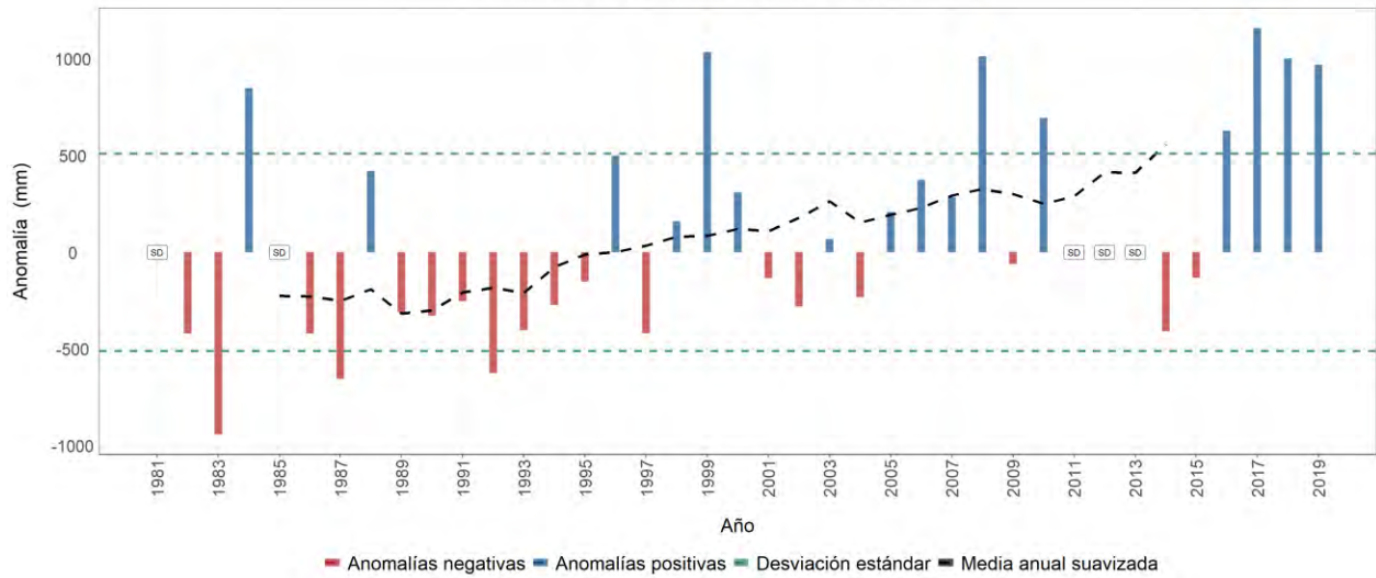
Estación meteorológica 2617034 - LA ORIENTAL, Quinchía, Risaralda Evolución anual de la anomalía de precipitación Promedio del período base (1981-2010): 2141 mm
