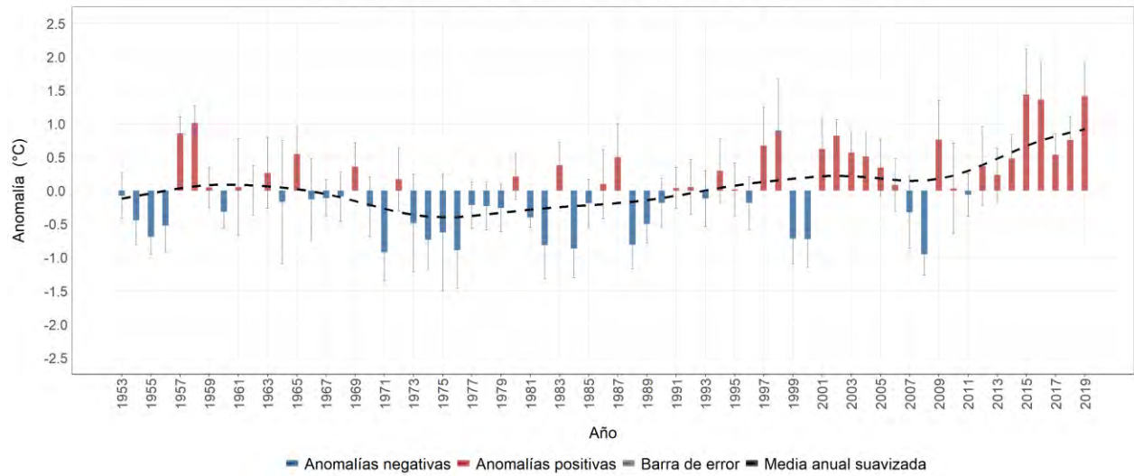
Estación meteorológica 2603506 - MANUEL MEJÍA, El Tambo, Cauca Evolución anual de la anomalía de temperatura máxima media Promedio del período base (1981-2010): 24.1 °C
