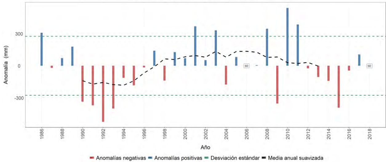
Estación meteorológica 2319049 - COCAL, Rionegro, Santander Evolución anual de la anomalía de precipitación Promedio del periodo base (1981-2010): 1370 mm
