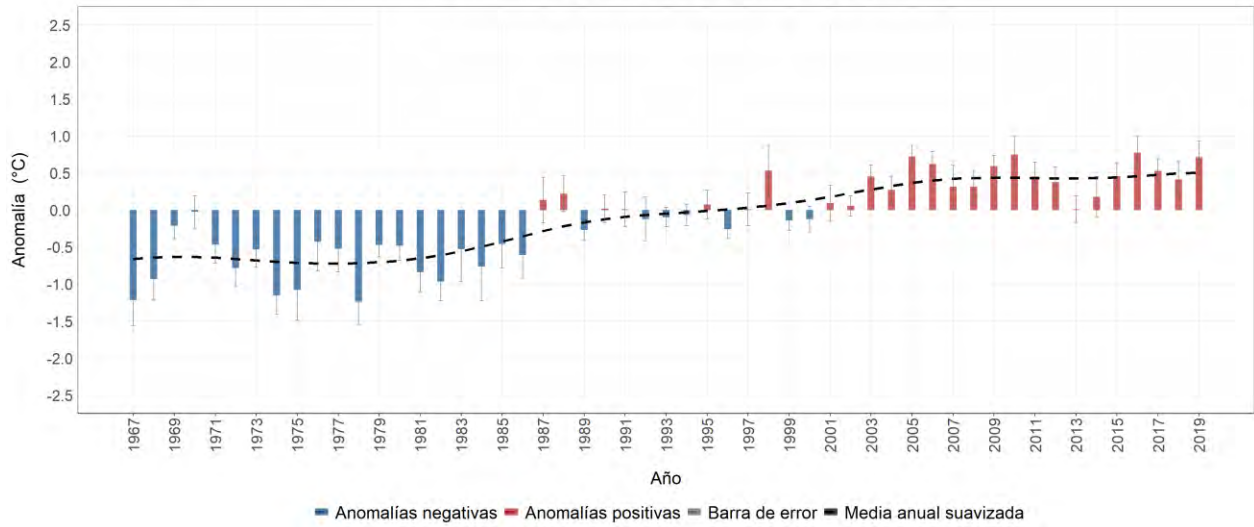
Estación meteorológica 2612510 - ARTURO GÓMEZ, Alcalá, Valle del Cauca Evolución anual de la anomalía de temperatura mínima media Promedio del período base (1981-2010): 16.9 °C
