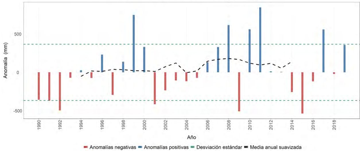
Estación meteorológica 2610512 - LA SIRENA, Sevilla, Valle del Cauca Evolución anual de la anomalía de precipitación Promedio del periodo base (1981-2010): 2112 mm
