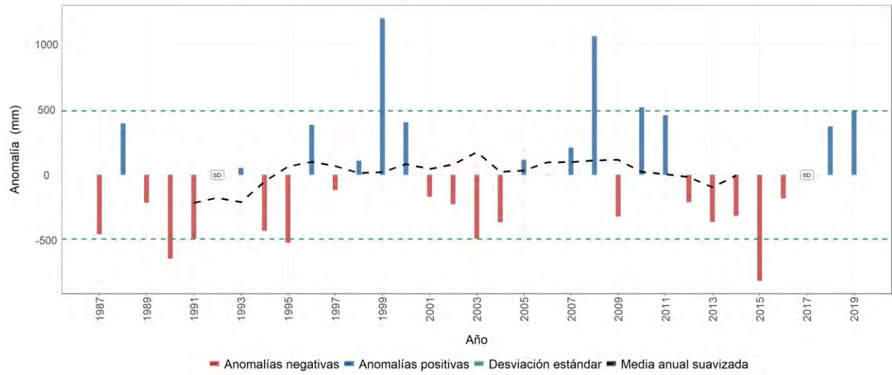
Estación meteorológica 2612068 - EL RECREO, Ulloa, Valle del Cauca Evolución anual de la anomalía de precipitación Promedio del período base (1981-2010): 2360 mm
