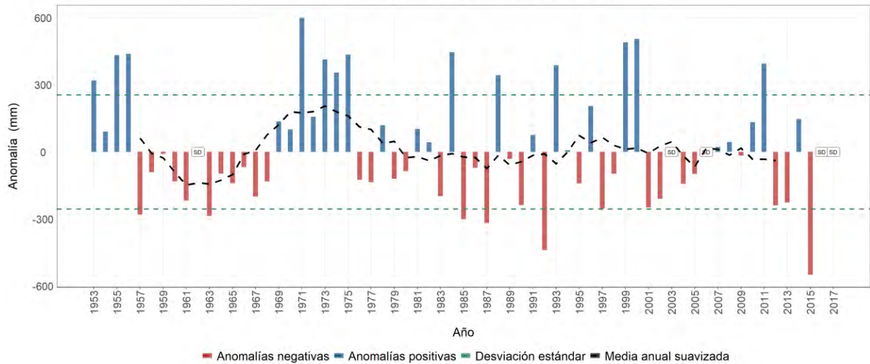
Estación meteorológica 5205507 - OSPINA PÉREZ, Consacá, Nariño Evolución anual de la anomalía de precipitación Promedio del periodo base (1981-2010): 1414 mm
