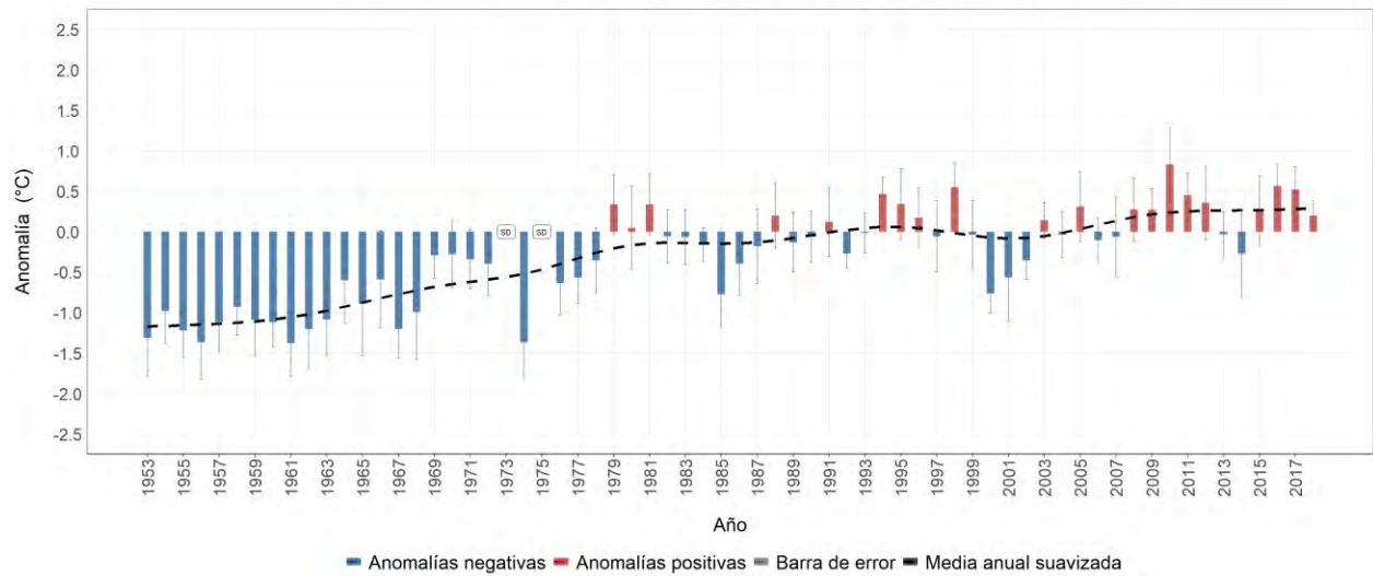
Estación meteorológica 2401502 - BERTHA, Moniquirá, Boyacá Evolución anual de la anomalía de temperatura mínima media Promedio del período base (1981-2010): 13.5 °C
