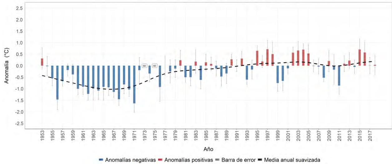
Estación meteorológica 2401502 - BERTHA, Moniquirá, Boyacá Evolución anual de la anomalía de temperatura máxima media Promedio del período base (1981-2010): 26.4 °C
