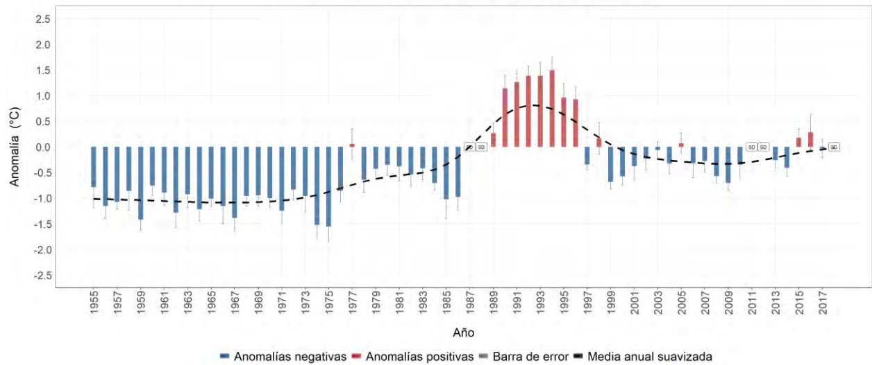
Estación meteorológica 2121507 - CHAPETÓN, Ibagué, Tolima Evolución anual de la anomalía de temperatura mínima media Promedio del periodo base (1981-2010): 16.9 °C
