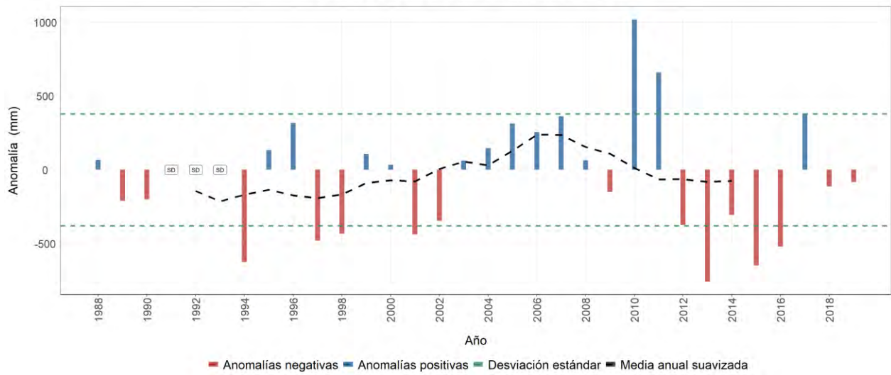
Estación meteorológica 2405016 - CASA DE TEJA, San Vicente De Chucurí, Santander Evolución anual de la anomalía de precipitación Promedio del periodo base (1981-2010): 2602 mm
