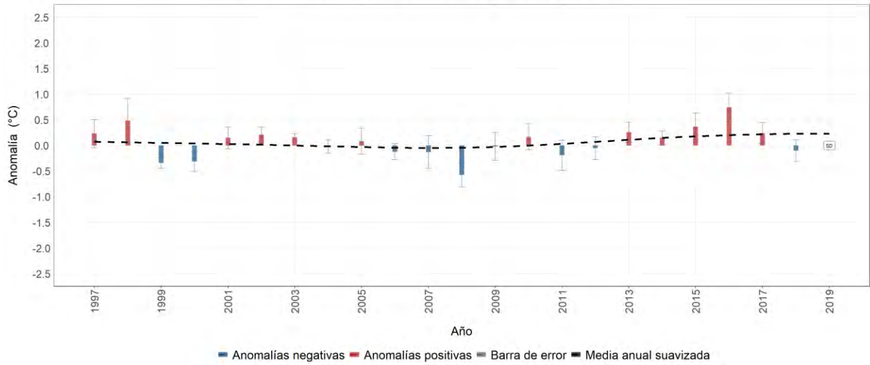
Estación meteorológica 8888884 - COCORNÁ, Cocorná, Antioquia Evolución anual de la anomalía de temperatura mínima media Promedio del período base (1981-2010): 17.3 °C
