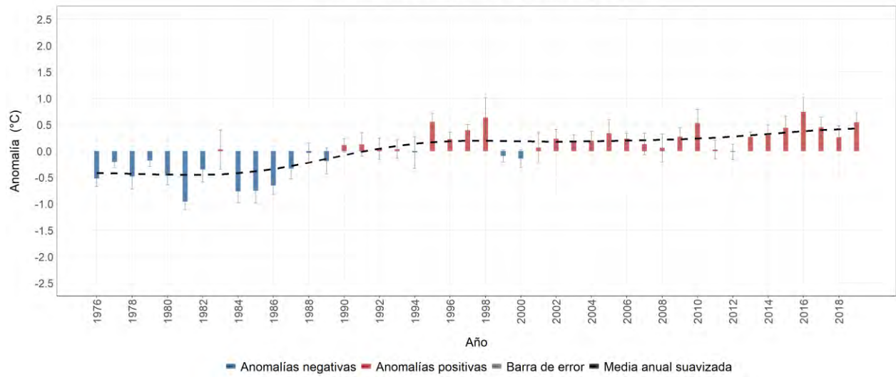
Estación meteorológica 2125513 - LA TRINIDAD, Líbano, Tolima Evolución anual de la anomalía de temperatura mínima media Promedio del período base (1981-2010): 16.4 °C
