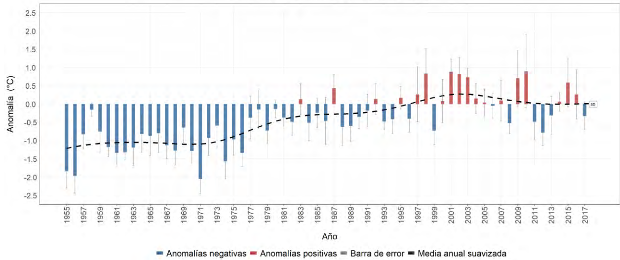
Estación meteorológica 2106503 - JORGE VILLAMIL, Gigante, Huila Evolución anual de la anomalía de temperatura máxima media Promedio del periodo base (1981-2010): 25 °C
