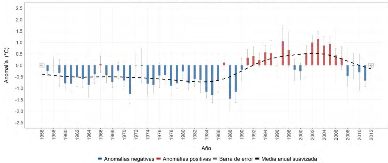
Estación meteorológica 2619501 - MIGUEL VALENCIA, Jardín, Antioquia Evolución anual de la anomalía de temperatura máxima media Promedio del período base (1981-2010): 25.9 °C
