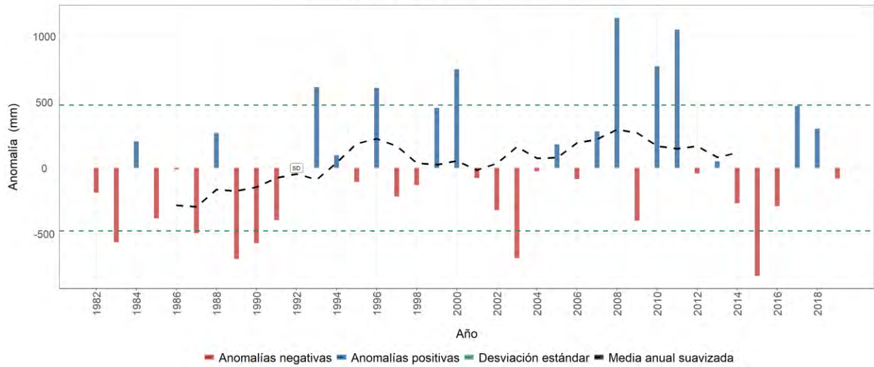
Estación meteorológica 2612056 - MÓNACO, Córdoba, Quindío Evolución anual de la anomalía de precipitación Promedio del período base (1981-2010): 2285 mm
