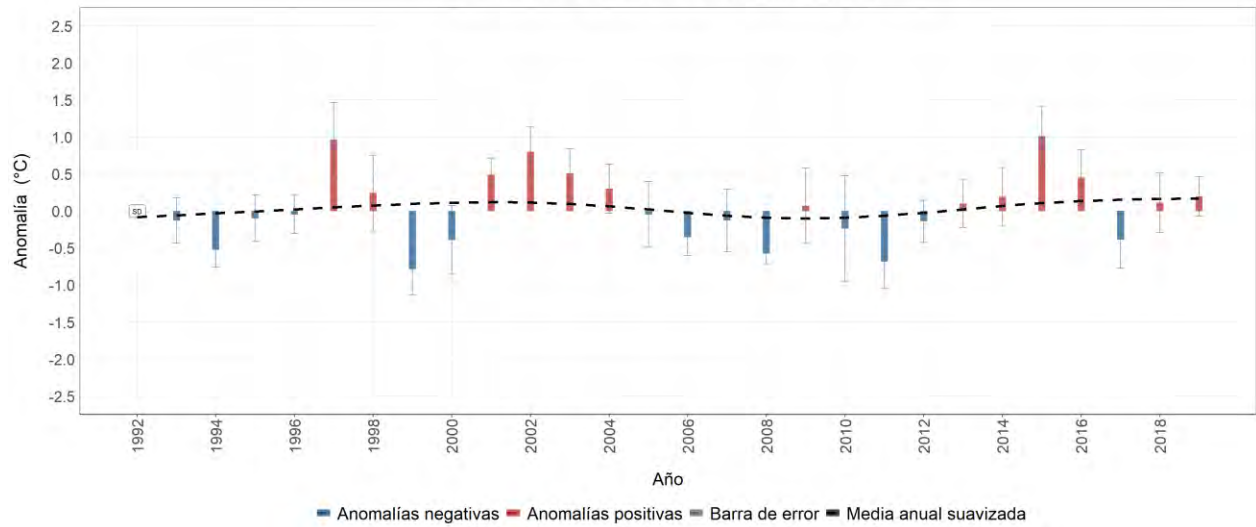
Estación meteorológica 2319519 - SAN ANTONIO, Floridablanca, Santander Evolución anual de la anomalía de temperatura máxima media Promedio del período base (1981-2010): 23.8 °C
