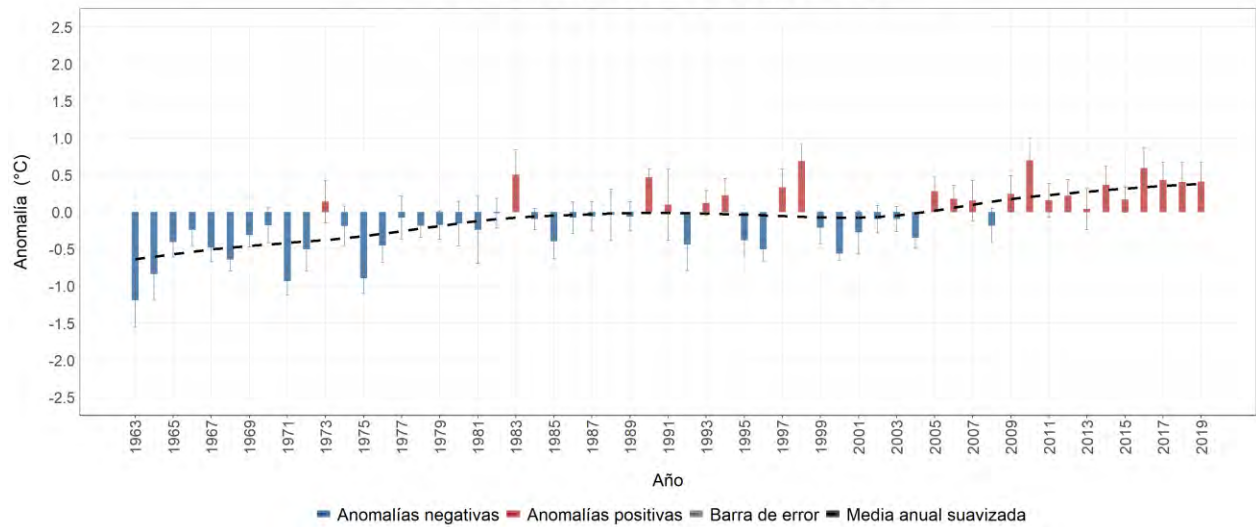
Estación meteorológica 2612508 - PARAGUAICITO, Buenavista, Quindío Evolución anual de la anomalía de temperatura mínima media Promedio del período base (1981-2010): 17.1 °C
