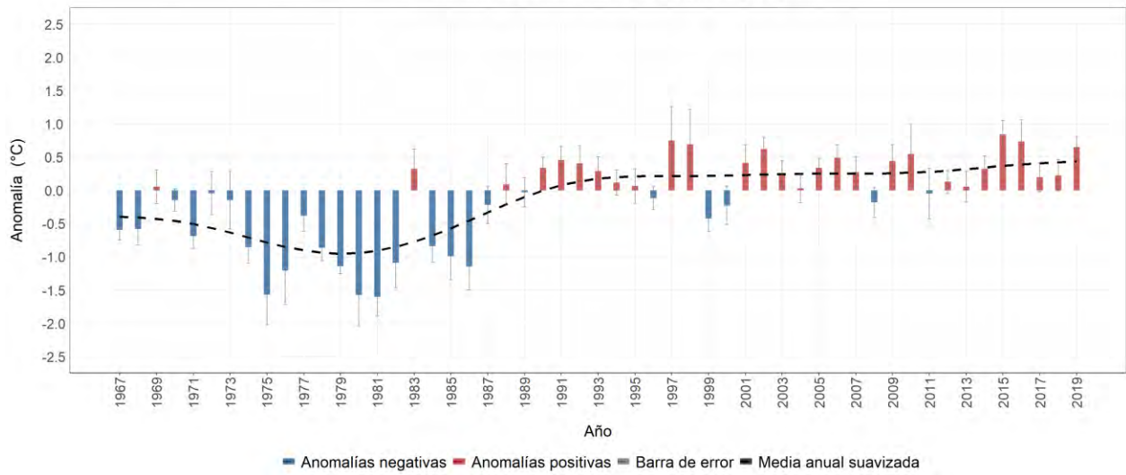
Estación meteorológica 2620502 - EL ROSARIO, Venecia, Antioquia Evolución anual de la anomalía de temperatura mínima media Promedio del periodo base (1981-2010): 16.4 °C
