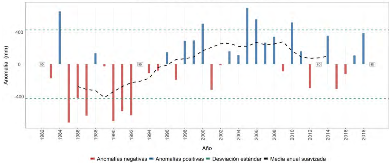
Estación meteorológica 2124006 - TOTARITO, Alvarado, Tolima Evolución anual de la anomalía de precipitación Promedio del periodo base (1981-2010): 1864 mm
