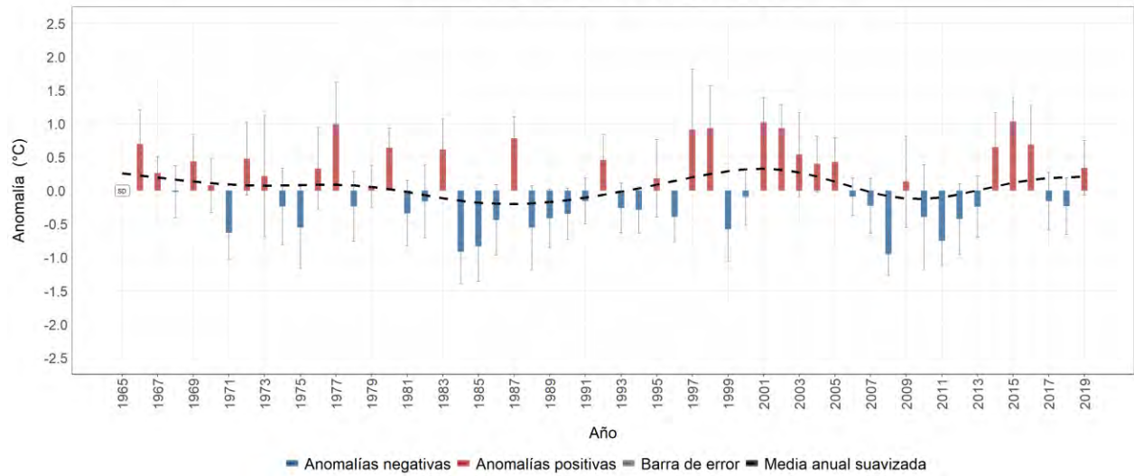
Estación meteorológica 2615509 - SANTÁGUEDA, Palestina, Caldas Evolución anual de la anomalía de temperatura máxima media Promedio del período base (1981-2010): 29.6 °C
