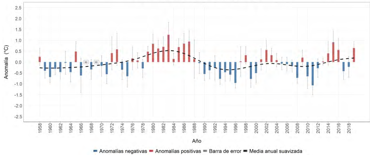
Estación meteorológica 2804501 - PUEBLO BELLO, Valledupar, Cesar Evolución anual de la anomalía de temperatura máxima media Promedio del período base (1981-2010): 27.2 °C
