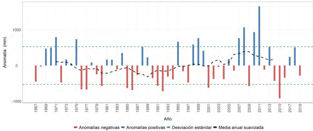
Estación meteorológica 2620502 - EL ROSARIO, Venecia, Antioquia Evolución anual de la anomalía de precipitación Promedio del periodo base (1981-2010): 2608 mm
