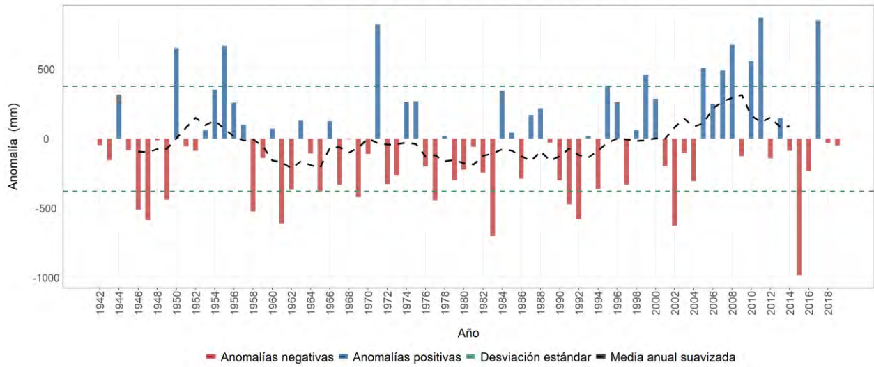
Estación meteorológica 2615502 - CENICAFÉ, Chinchiná, Caldas Evolución anual de la anomalía de precipitación Promedio del período base (1981-2010): 2599 mm
