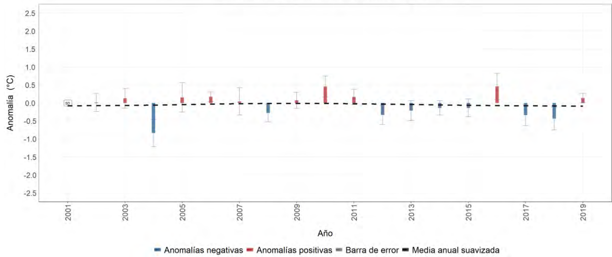
Estación meteorológica 742 - EL ROBLE, Los Santos, Santander Evolución anual de la anomalía de temperatura mínima media Promedio del período base (1981-2010): 14.6 °C
