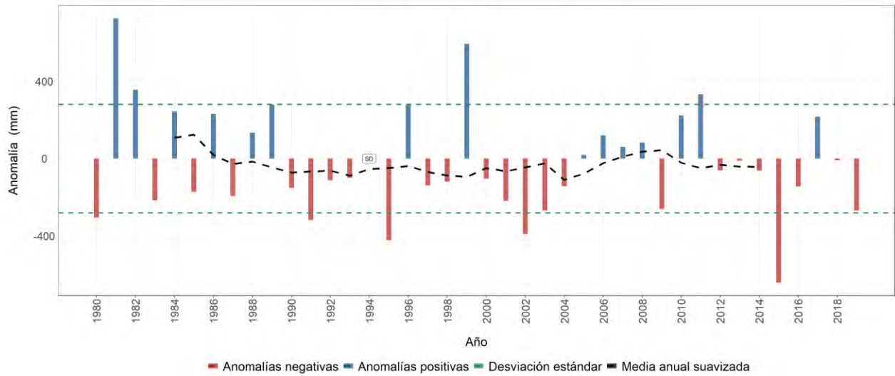
Estación meteorológica 2609501 - LA SELVA, Ginebra, Valle del Cauca Evolución anual de la anomalía de precipitación Promedio del periodo base (1981-2010): 1652 mm
