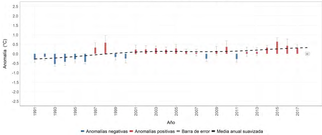
Estación meteorológica 2120608 - MESITAS DE SANTA INÉS, Cachipay, Cundinamarca Evolución anual de la anomalía de temperatura mínima media Promedio del período base (1981-2010): 17.5 °C
