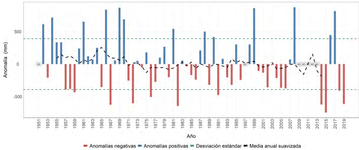
Estación meteorológica 2 - LA VICTORIA, Santa Marta, Magdalena Evolución anual de la anomalía de precipitación Promedio del periodo base (1981-2010): 2417 mm
