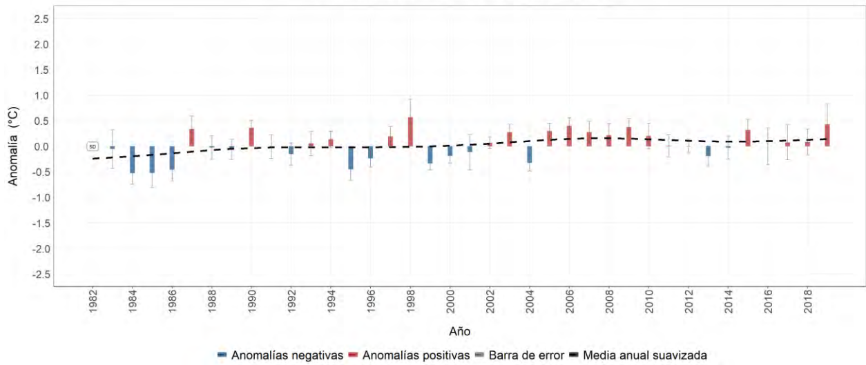
Estación meteorológica 2612525 - MARACAY, Quimbaya, Quindío Evolución anual de la anomalía de temperatura mínima media Promedio del período base (1981-2010): 16.3 °C
