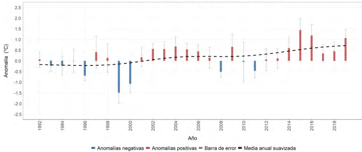
Estación meteorológica 2610512 - LA SIRENA, Sevilla, Valle del Cauca Evolución anual de la anomalía de temperatura máxima media Promedio del período base (1981-2010): 25.3 °C
