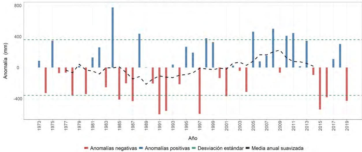
Estación meteorológica 2125513 - LA TRINIDAD, Líbano, Tolima Evolución anual de la anomalía de precipitación Promedio del periodo base (1981-2010): 2203 mm
