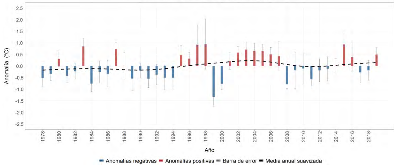
Estación meteorológica 2120607 - MISIONES, El Colegio, Cundinamarca Evolución anual de la anomalía de temperatura máxima media Promedio del período base (1981-2010): 23.8 °C
