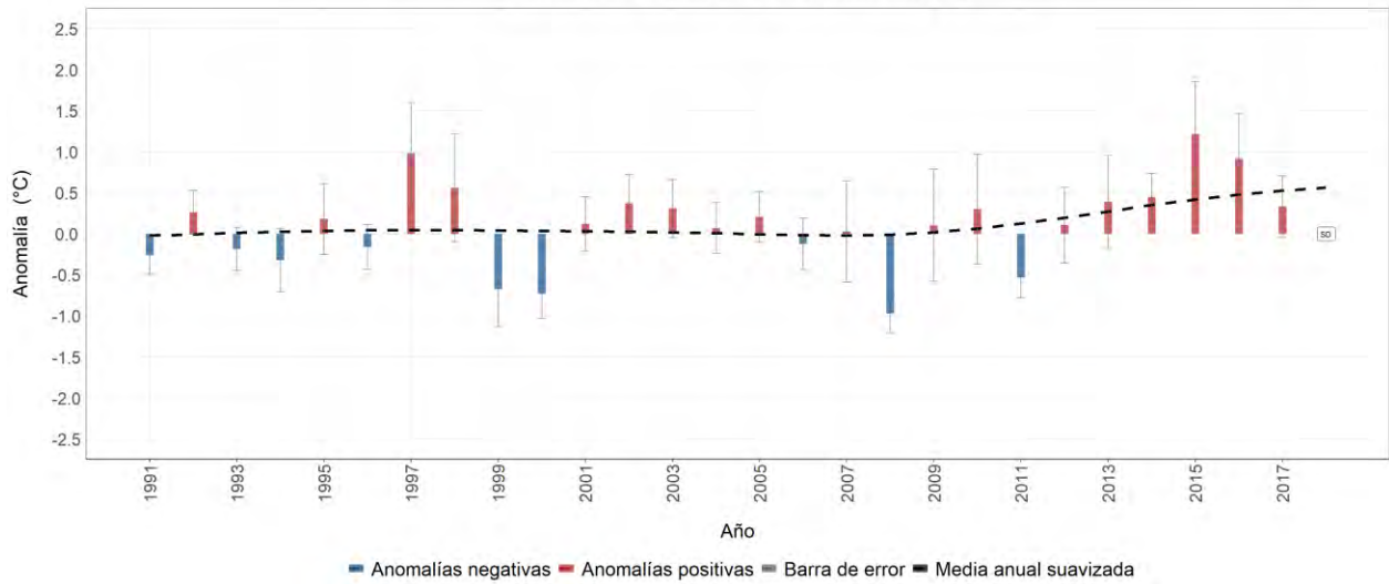
Estación meteorológica 2120608 - MESITAS DE SANTA INÉS, Cachipay, Cundinamarca Evolución anual de la anomalía de temperatura máxima media Promedio del período base (1981-2010): 25.2 °C
