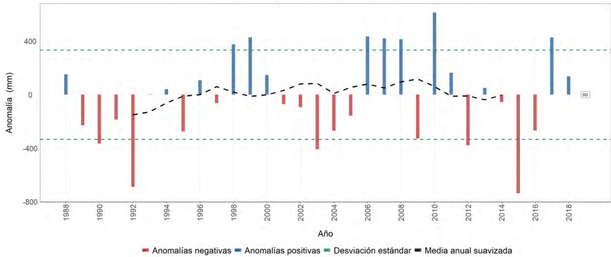
Estación meteorológica 2612067 - EL BERRIÓN, Cartago, Valle del Cauca Evolución anual de la anomalía de precipitación Promedio del periodo base (1981-2010): 1853 mm
