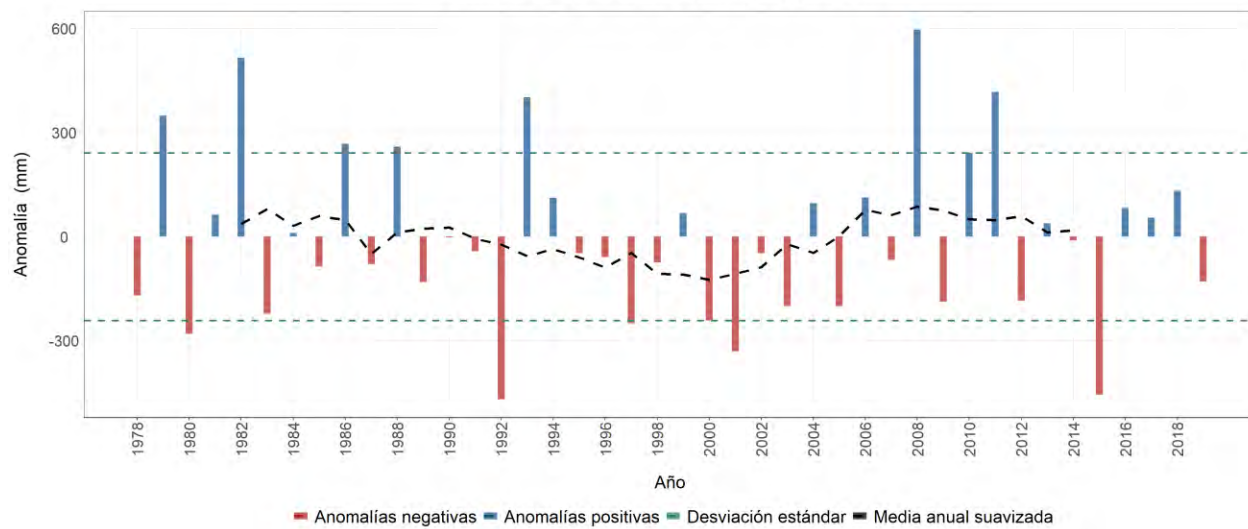
Estación meteorológica 2120607 - MISIONES, El Colegio, Cundinamarca Evolución anual de la anomalía de precipitación Promedio del periodo base (1981-2010): 1421 mm
