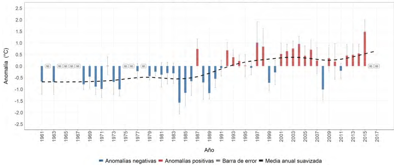
Estación meteorológica 2613507 - EL CEDRAL, Pereira, Risaralda Evolución anual de la anomalía de temperatura máxima media Promedio del periodo base (1981-2010): 20 °C
