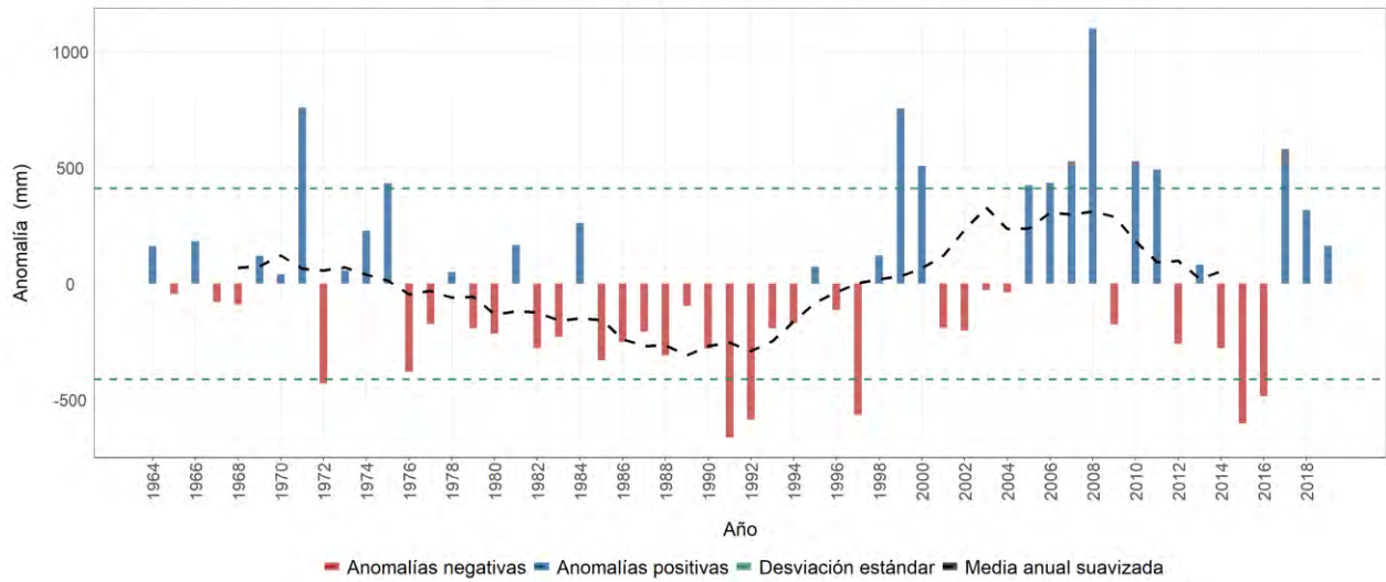
Estación meteorológica 2615509 - SANTÁGUEDA, Palestina, Caldas Evolución anual de la anomalía de precipitación Promedio del período base (1981-2010): 2276 mm
