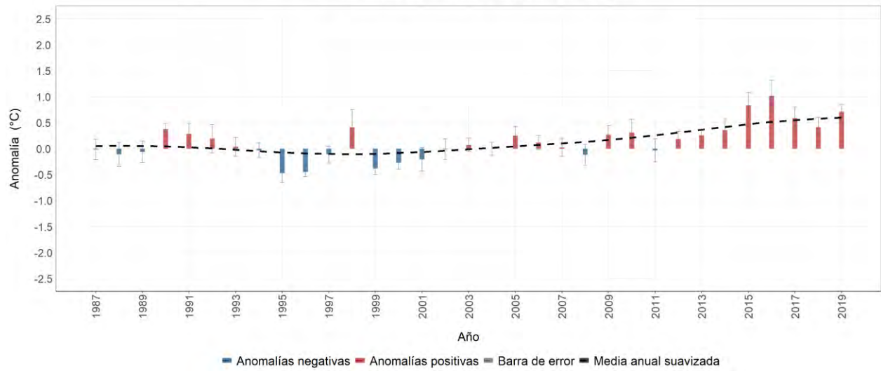
Estación meteorológica 2612524 - LA CATALINA, Pereira, Risaralda Evolución anual de la anomalía de temperatura mínima media Promedio del período base (1981-2010): 17.2 °C
