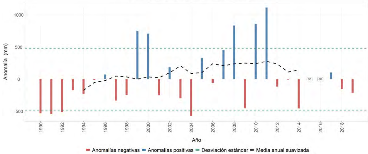
Estación meteorológica 2612057 - EL PORVENIR, Pijao, Quindío Evolución anual de la anomalía de precipitación Promedio del período base (1981-2010): 2078 mm
