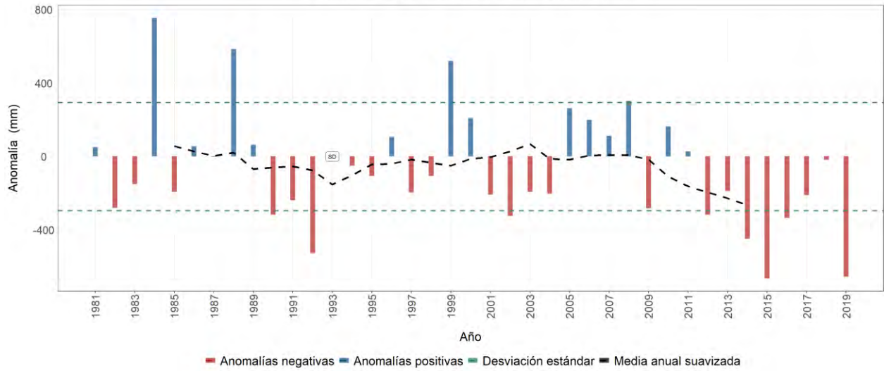
Estación meteorológica 2614030 - BUENOS AIRES, Guática, Risaralda Evolución anual de la anomalía de precipitación Promedio del período base (1981-2010): 1814 mm
