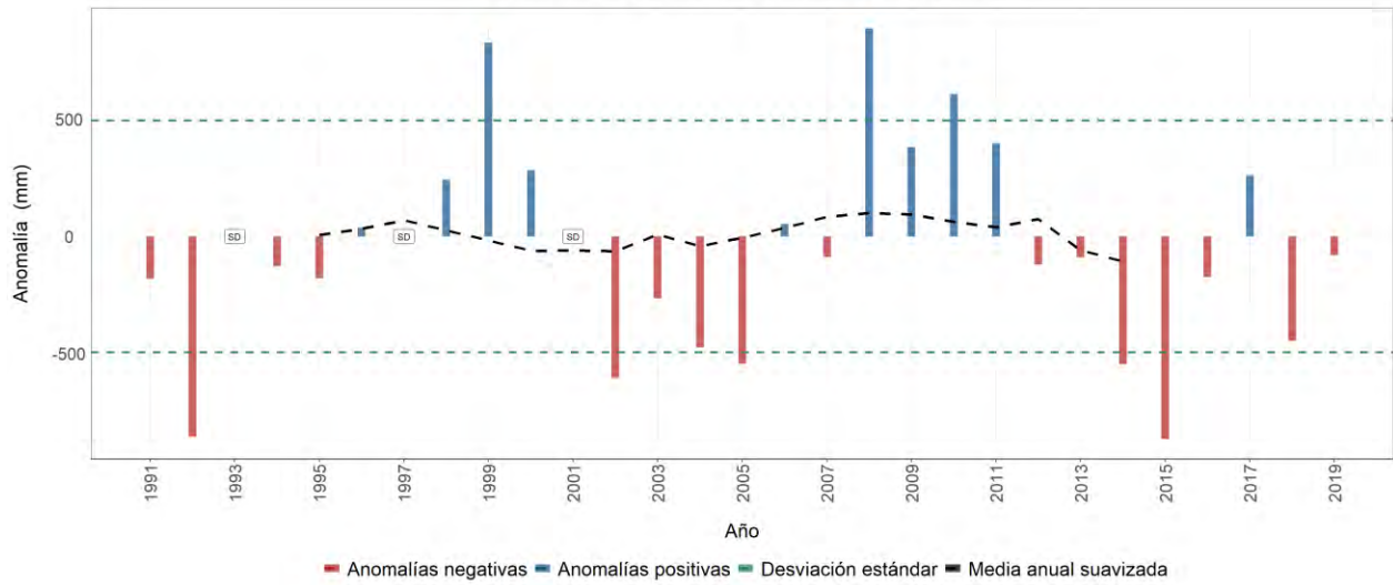
Estación meteorológica 2207004 - EL RECREO, Ortega, Tolima Evolución anual de la anomalía de precipitación Promedio del periodo base (1981-2010): 3023 mm
