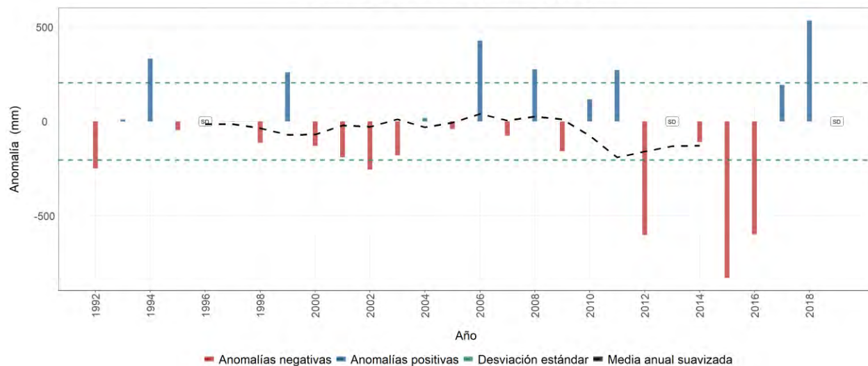
Estación meteorológica 2119043 - SAN LUIS, Arbeláez, Cundinamarca Evolución anual de la anomalía de precipitación Promedio del período base (1981-2010): 1438 mm
