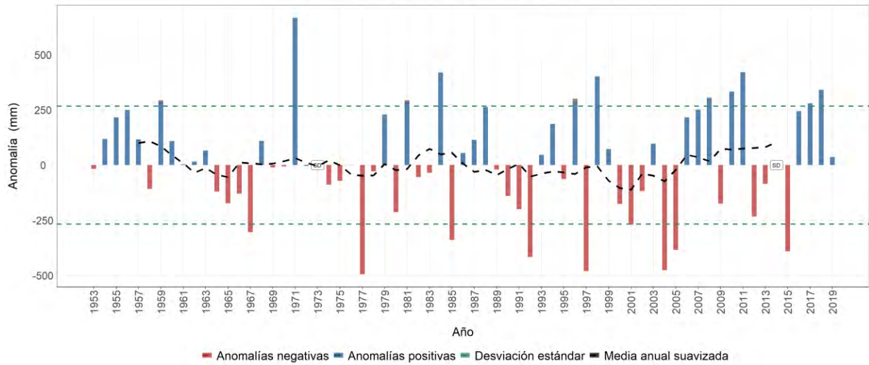
Estación meteorológica 2401502 - BERTHA, Moniquirá, Boyacá Evolución anual de la anomalía de precipitación Promedio del periodo base (1981-2010): 1988 mm
