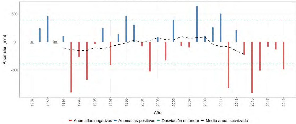
Estación meteorológica 2613044 - LA PALMA, Palestina, Caldas Evolución anual de la anomalía de precipitación Promedio del periodo base (1981-2010): 2734 mm
