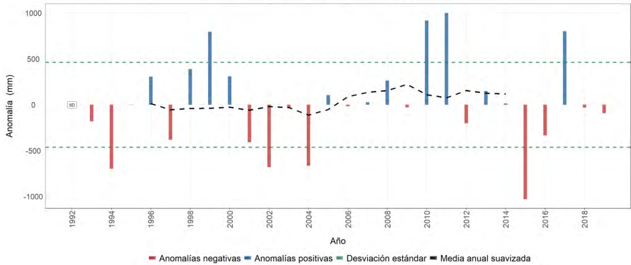
Estación meteorológica 2615038 - LA DIVISA, Chinchiná, Caldas Evolución anual de la anomalía de precipitación Promedio del período base (1981-2010): 2845 mm
