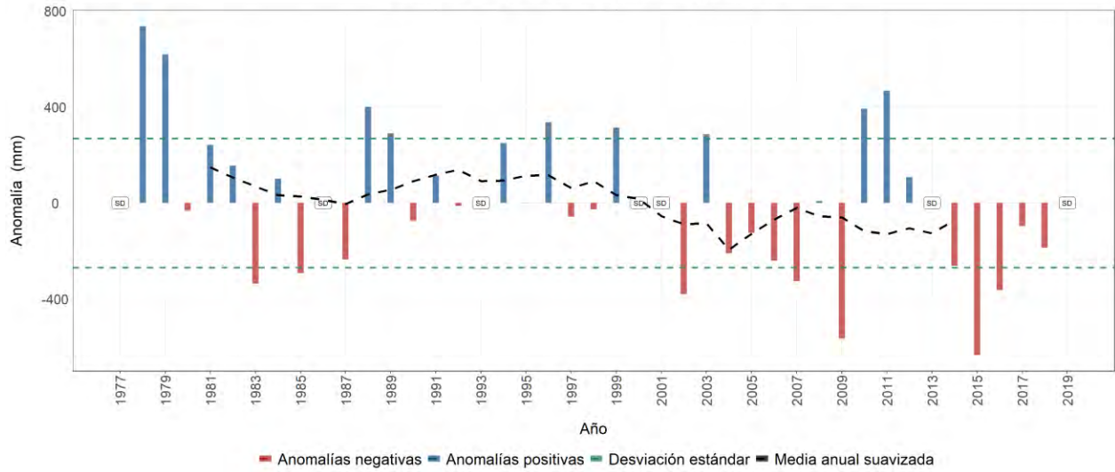
Estación meteorológica 2319062 - LOS COCOS, Rionegro, Santander Evolución anual de la anomalía de precipitación Promedio del periodo base (1981-2010): 1682 mm
