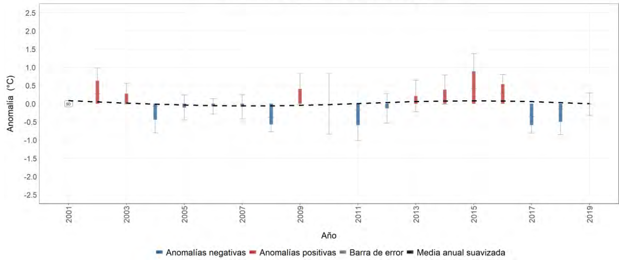
Estación meteorológica 742 - EL ROBLE, Los Santos, Santander Evolución anual de la anomalía de temperatura máxima media Promedio del período base (1981-2010): 24.8 °C
