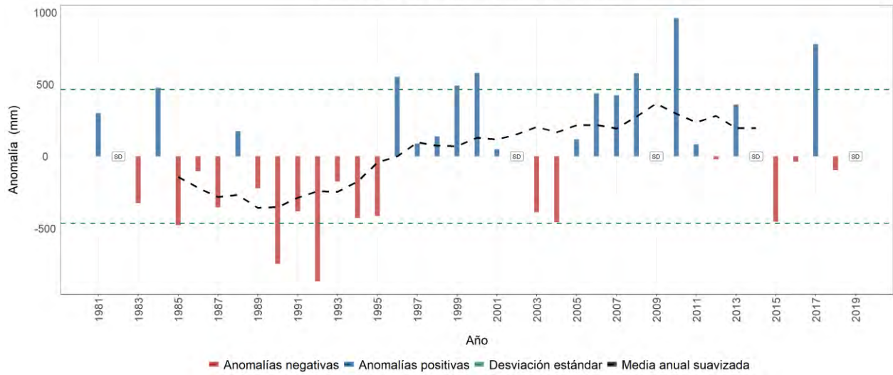
Estación meteorológica 2613051 - COMBIA, Pereira, Risaralda Evolución anual de la anomalía de precipitación Promedio del periodo base (1981-2010): 2268 mm
