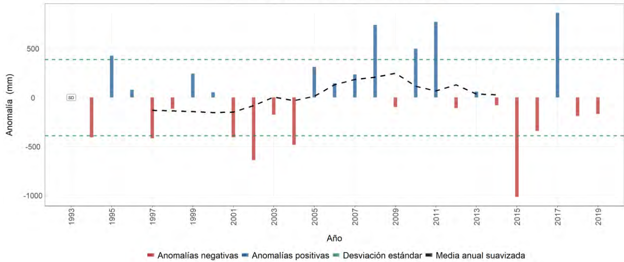
Estación meteorológica 37 - PLANALTO, Manizales, Caldas Evolución anual de la anomalía de precipitación Promedio del período base (1981-2010): 2588 mm
