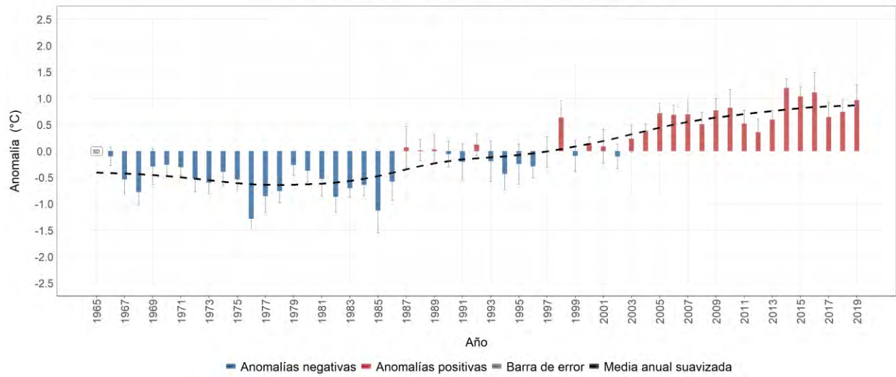
Estación meteorológica 2615509 - SANTÁGUEDA, Palestina, Caldas Evolución anual de la anomalía de temperatura mínima media Promedio del período base (1981-2010): 18 °C
