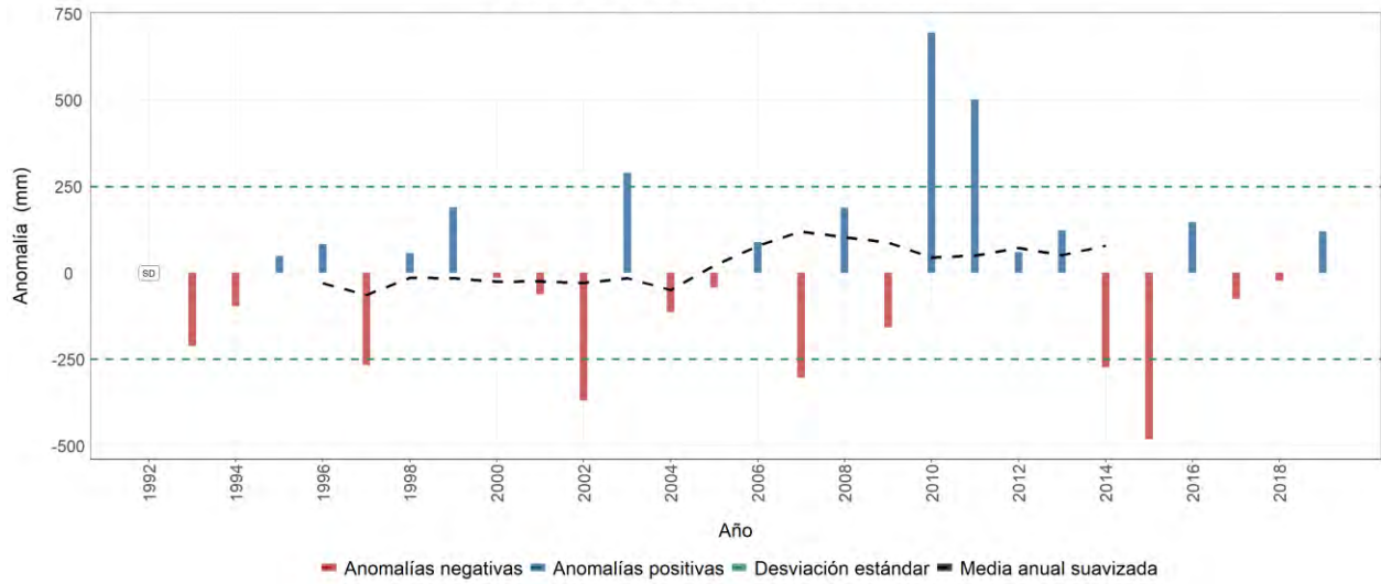
Estación meteorológica 2319519 - SAN ANTONIO, Floridablanca, Santander Evolución anual de la anomalía de precipitación Promedio del período base (1981-2010): 1524 mm
