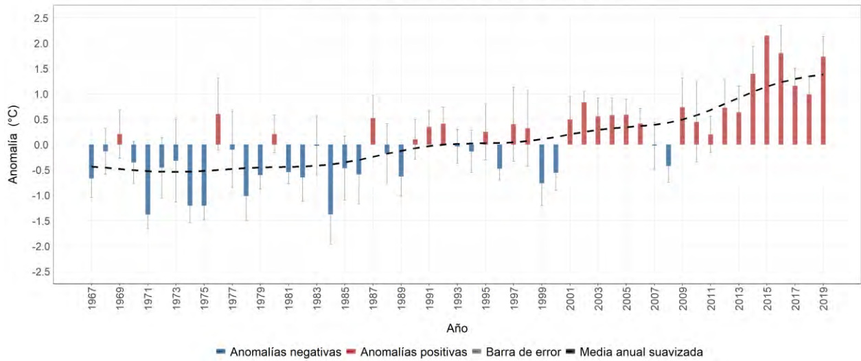
Estación meteorológica 2612510 - ARTURO GÓMEZ, Alcalá, Valle del Cauca Evolución anual de la anomalía de temperatura máxima media Promedio del período base (1981-2010): 27.6 °C
