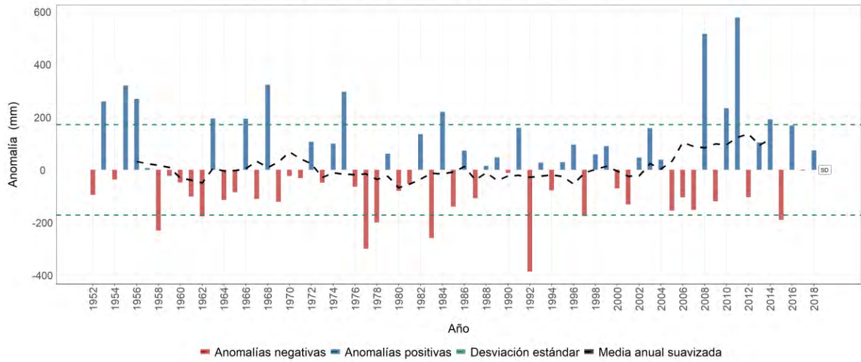
Estación meteorológica 2119503 - GRANJA TIBACUY, Tibacuy, Cundinamarca Evolución anual de la anomalía de precipitación Promedio del periodo base (1981-2010): 1099 mm
