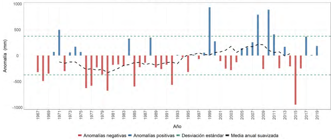
Estación meteorológica 2612510 - ARTURO GÓMEZ, Alcalá, Valle del Cauca Evolución anual de la anomalía de precipitación Promedio del período base (1981-2010): 2080 mm
