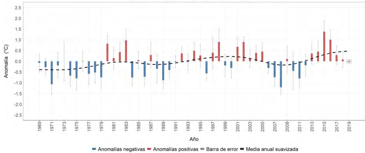
Estación meteorológica 2608511 - MANUEL M. MALLARINO, Trujillo, Valle del Cauca Evolución anual de la anomalía de temperatura máxima media Promedio del período base (1981-2010): 26.3 °C
