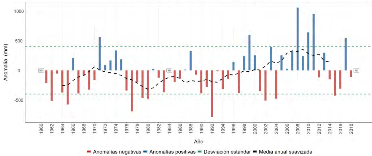
Estación meteorológica 2613506 - EL JAZMÍN, Santa Rosa De Cabal, Risaralda Evolución anual de la anomalía de precipitación Promedio del período base (1981-2010): 2716 mm
