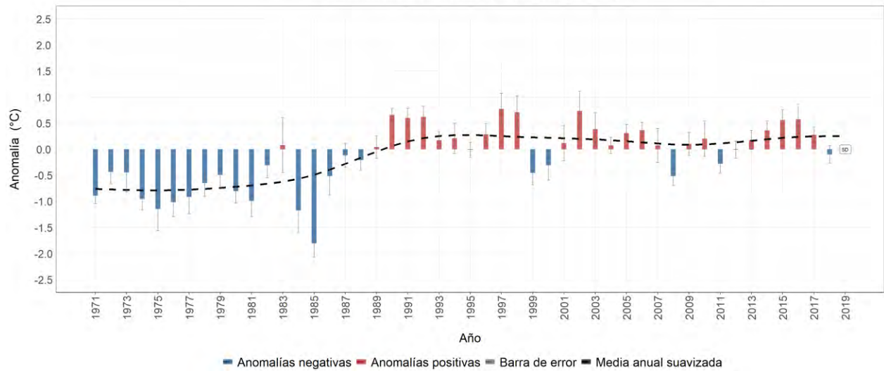
Estación meteorológica 2306513 - MONTELÍBANO, Yacopi, Cundinamarca Evolución anual de la anomalía de temperatura mínima media Promedio del período base (1981-2010): 17.2 °C
