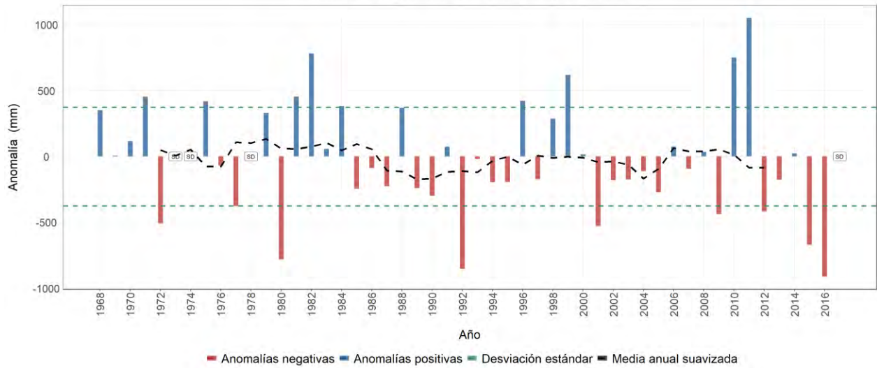
Estación meteorológica 2613507 - EL CEDRAL, Pereira, Risaralda Evolución anual de la anomalía de precipitación Promedio del período base (1981-2010): 2646 mm
