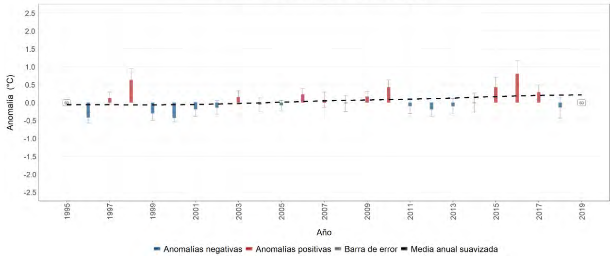
Estación meteorológica 741 - ALBERTO SANTOS, Socorro, Santander Evolución anual de la anomalía de temperatura mínima media Promedio del período base (1981-2010): 15.9 °C
