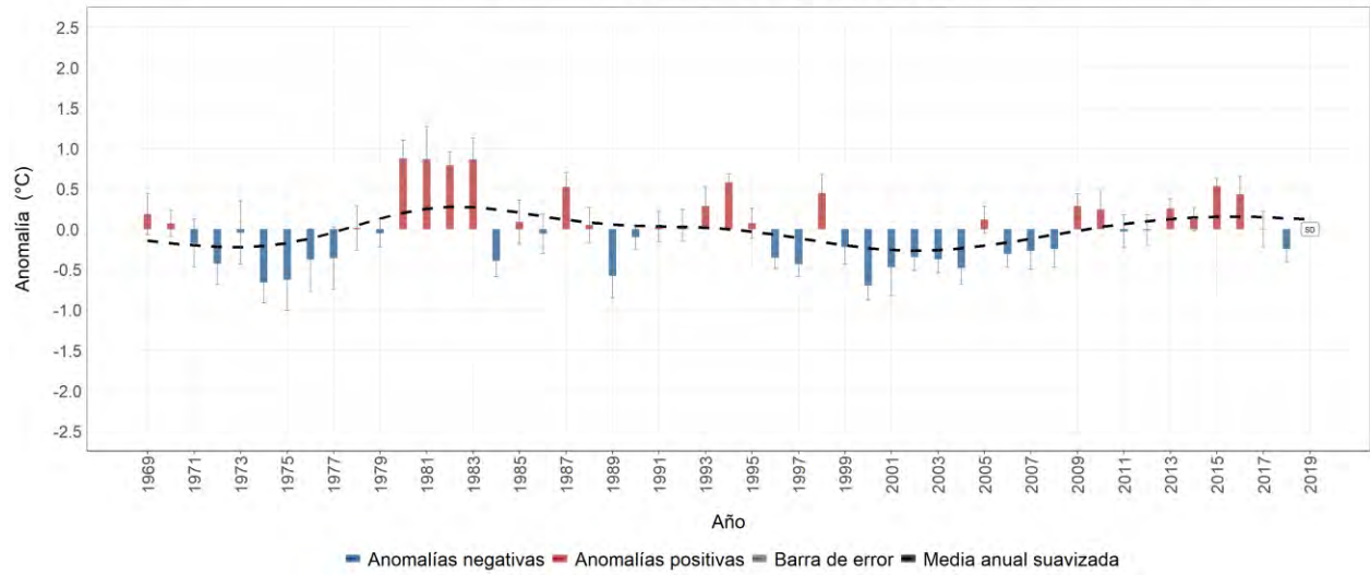
Estación meteorológica 2608511 - MANUEL M. MALLARINO, Trujillo, Valle del Cauca Evolución anual de la anomalía de temperatura mínima media Promedio del período base (1981-2010): 16.8 °C
