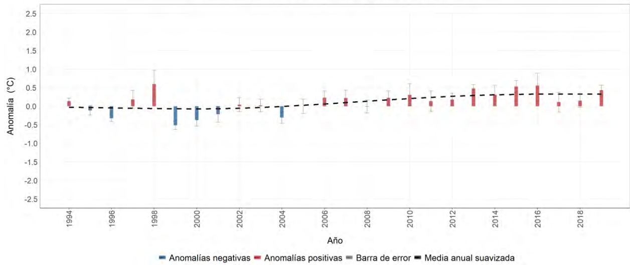
Estación meteorológica 37 - PLANALTO, Manizales, Caldas Evolución anual de la anomalía de temperatura mínima media Promedio del período base (1981-2010): 16.6 °C
