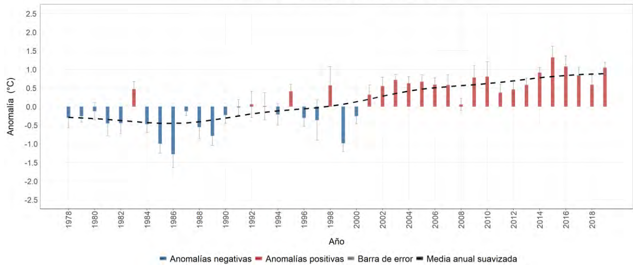
Estación meteorológica 2120607 - MISIONES, El Colegio, Cundinamarca Evolución anual de la anomalía de temperatura mínima media Promedio del período base (1981-2010): 17 °C
