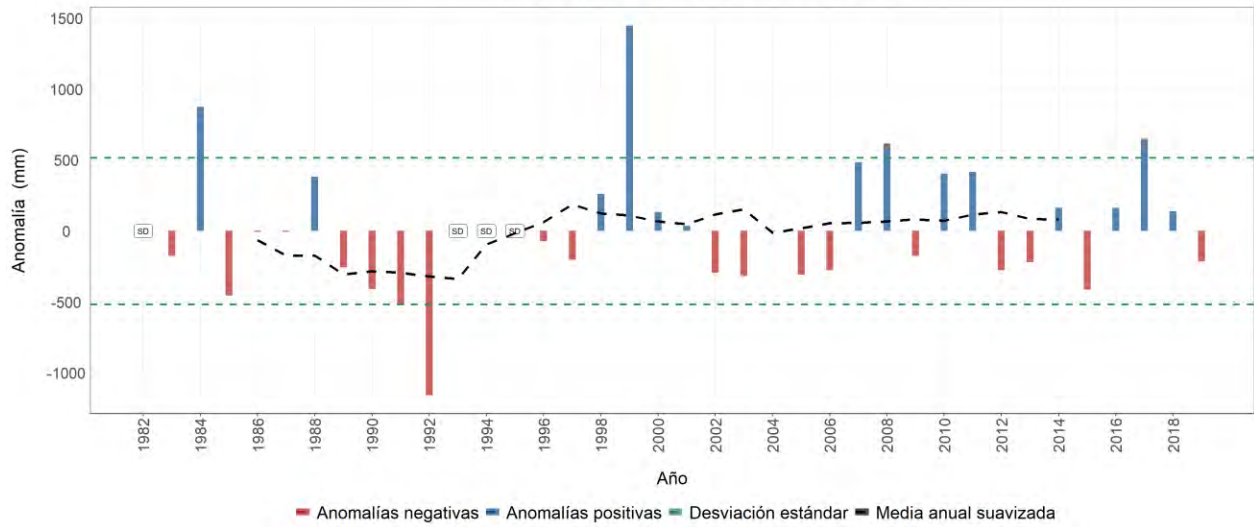
Estación meteorológica 2612024 - SORRENTO, Montenegro, Quindío Evolución anual de la anomalía de precipitación Promedio del período base (1981-2010): 2064 mm
