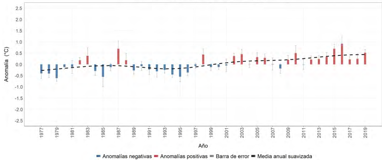
Estación meteorológica 2612507 - LA BELLA, Calarca, Quindío Evolución anual de la anomalía de temperatura mínima media Promedio del período base (1981-2010): 16.3 °C
