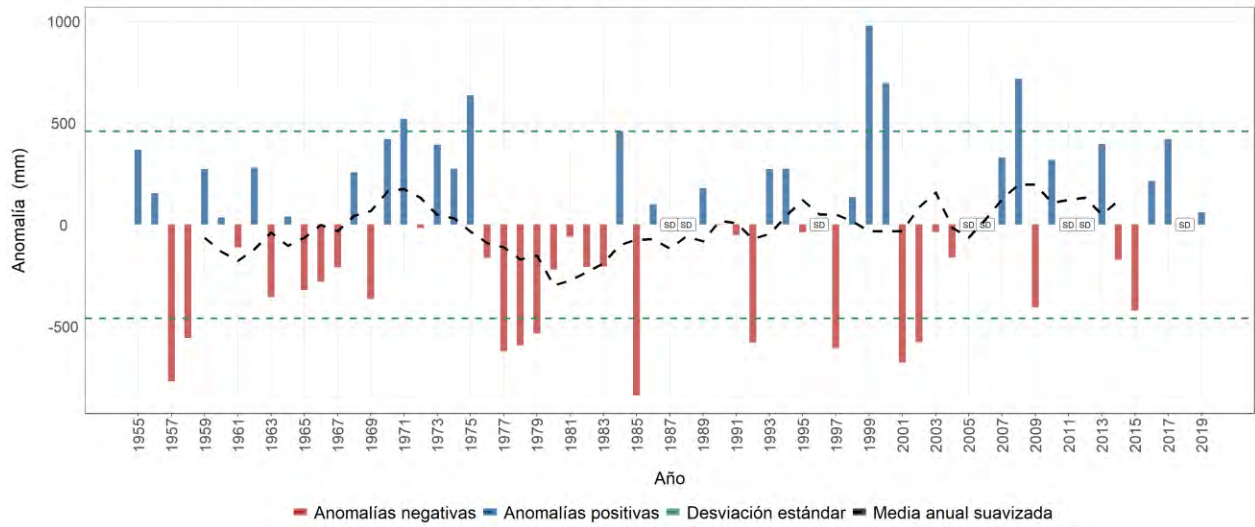
Estación meteorológica 2121507 - CHAPETÓN, Ibagué, Tolima Evolución anual de la anomalía de precipitación Promedio del periodo base (1981-2010): 2055 mm
