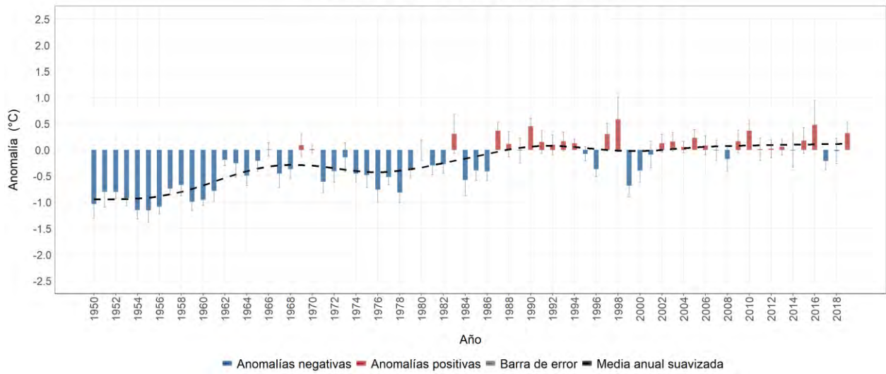
Estación meteorológica 2615502 - CENICAFÉ, Chinchiná, Caldas Evolución anual de la anomalía de temperatura mínima media Promedio del período base (1981-2010): 17 °C
