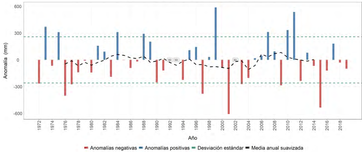
Estación meteorológica 5403004 - SANTIAGO GUTIÉRREZ, Argelia, Valle del Cauca Evolución anual de la anomalía de precipitación Promedio del período base (1981-2010): 1432 mm
