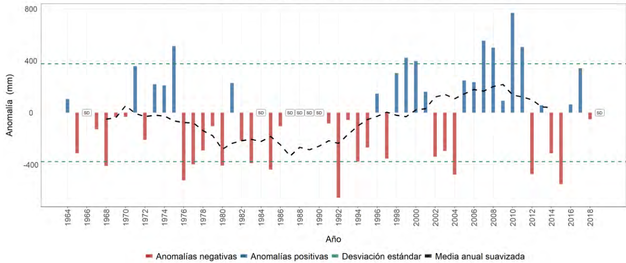
Estación meteorológica 2613021 - LOS CÁMBULOS, Pereira, Risaralda Evolución anual de la anomalía de precipitación Promedio del periodo base (1981-2010): 1934 mm
