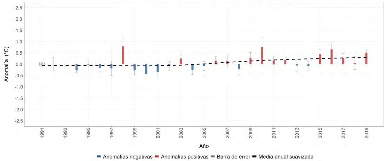
Estación meteorológica 1605511 - GABRIEL MARÍA BARRIGA, Convención, Norte de Santander Evolución anual de la anomalía de temperatura mínima media Promedio del período base (1981-2010): 17 °C
