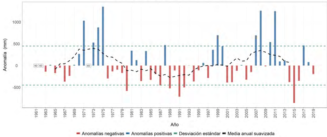
Estación meteorológica 2618005 - GUAYMARAL, Aguadas, Caldas Evolución anual de la anomalía de precipitación Promedio del período base (1981-2010): 1859 mm
