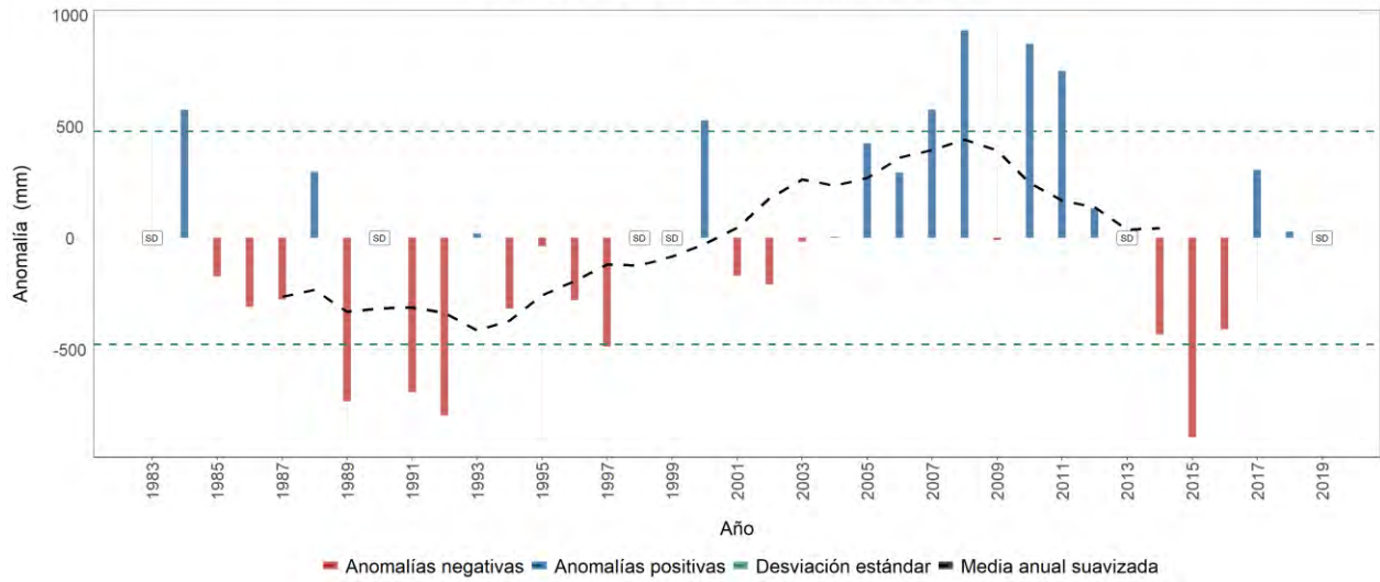
Estación meteorológica 2618004 - CUATRO ESQUINAS, Aguadas, Caldas Evolución anual de la anomalía de precipitación Promedio del periodo base (1981-2010): 1797 mm
