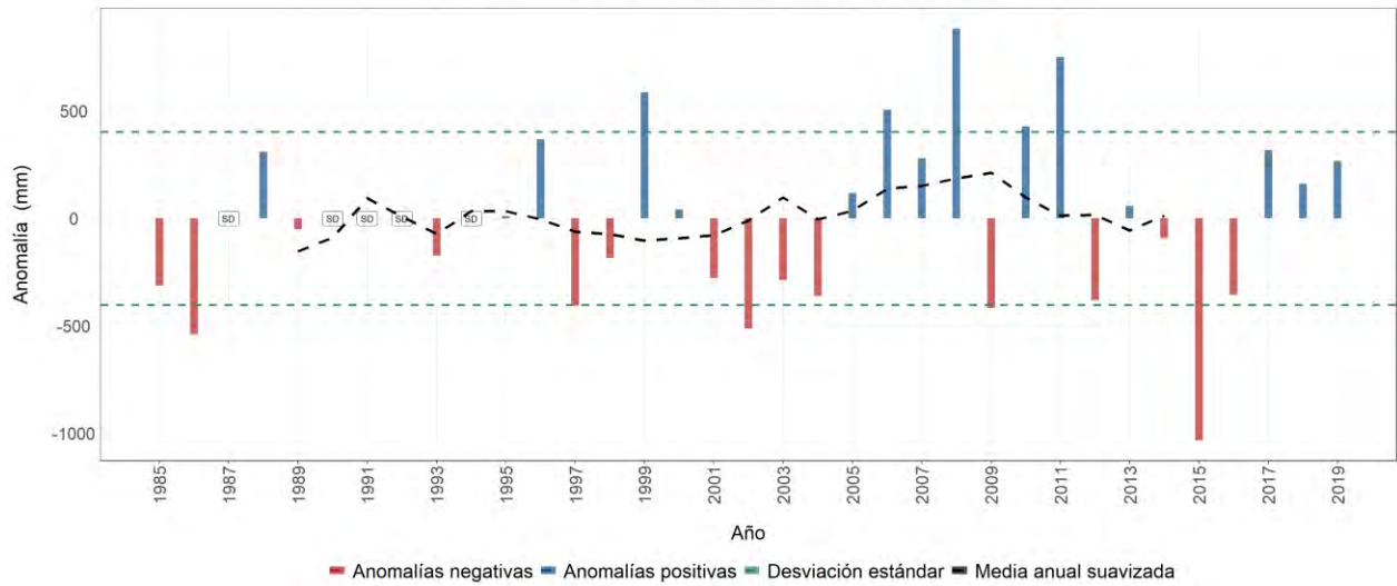
Estación meteorológica 2615020 - LA SELVA, Manizales, Caldas Evolución anual de la anomalía de precipitación Promedio del período base (1981-2010): 2414 mm
