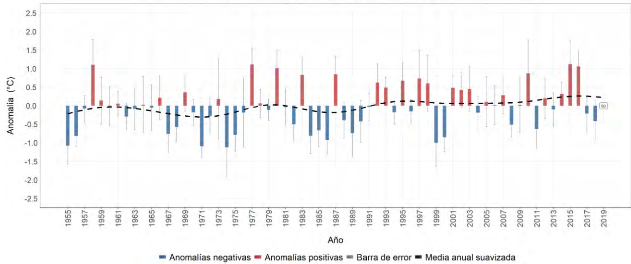
Estación meteorológica 1602506 - FRANCISCO ROMERO, Salazar, Norte de Santander Evolución anual de la anomalía de temperatura máxima media Promedio del período base (1981-2010): 27.9 °C
