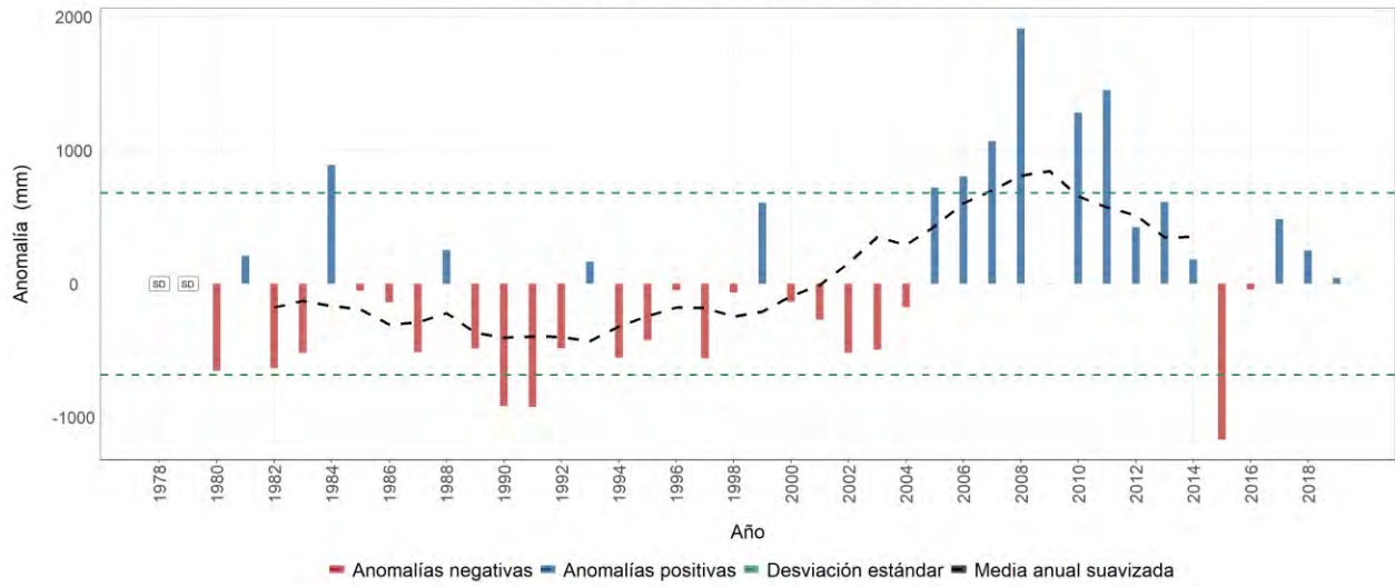
Estación meteorológica 2617032 - LA ARGENTINA, Riosucio, Caldas Evolución anual de la anomalía de precipitación Promedio del período base (1981-2010): 2657 mm
