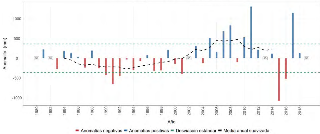
Estación meteorológica 2615035 - JAVA, Manizales, Caldas Evolución anual de la anomalía de precipitación Promedio del período base (1981-2010): 1982 mm
