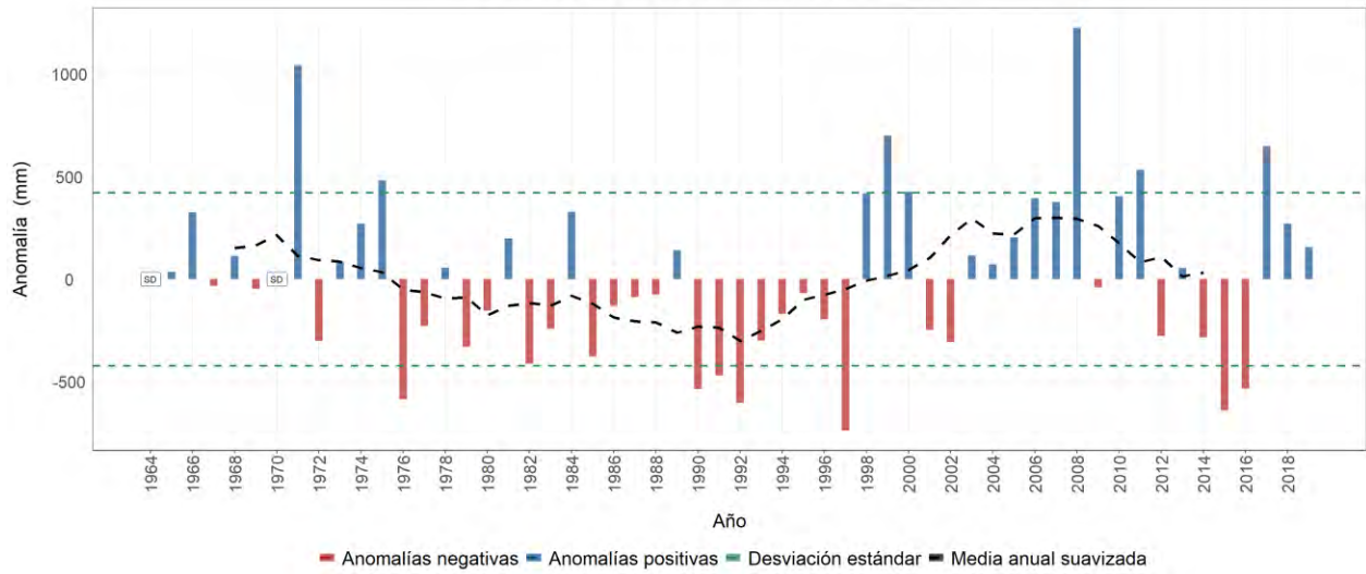
Estación meteorológica 2615514 - GRANJA LUKER, Palestina, Caldas Evolución anual de la anomalía de precipitación Promedio del período base (1981-2010): 2270 mm
