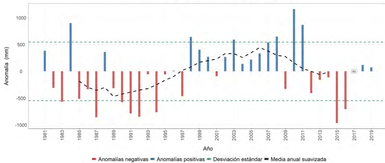
Estación meteorológica 2614020 - LA TRIBUNA, Balboa, Risaralda Evolución anual de la anomalía de precipitación Promedio del período base (1981-2010): 2359 mm
