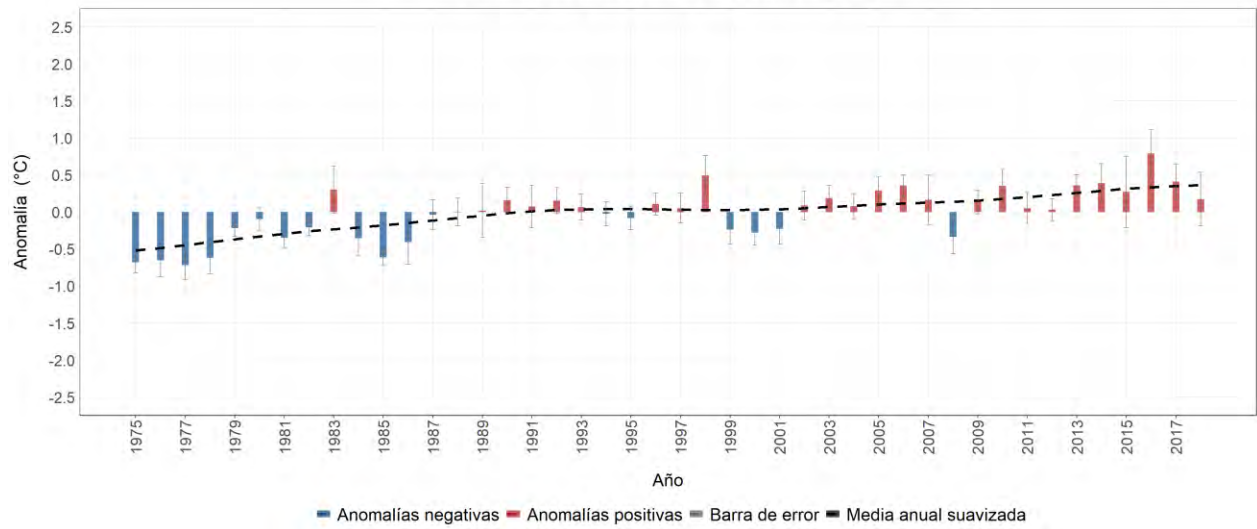
Estación meteorológica 5403503 - ALBÁN, El Cairo, Valle del Cauca Evolución anual de la anomalía de temperatura mínima media Promedio del período base (1981-2010): 15.7 °C
