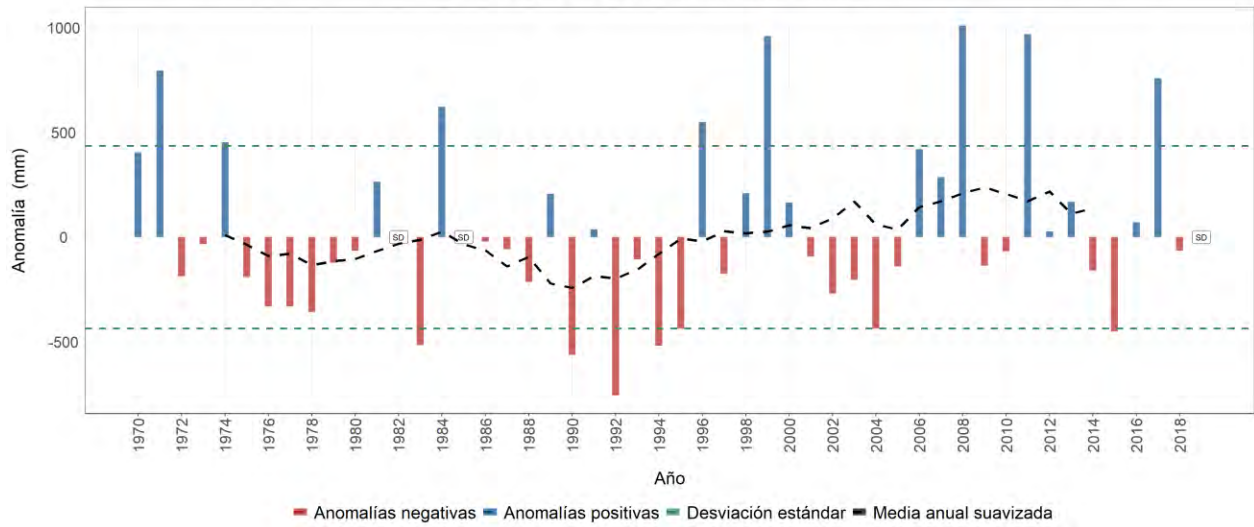
Estación meteorológica 2613023 - PLANTA DE TRATAMIENTO, Pereira, Risaralda Evolución anual de la anomalía de precipitación Promedio del periodo base (1981-2010): 2683 mm
