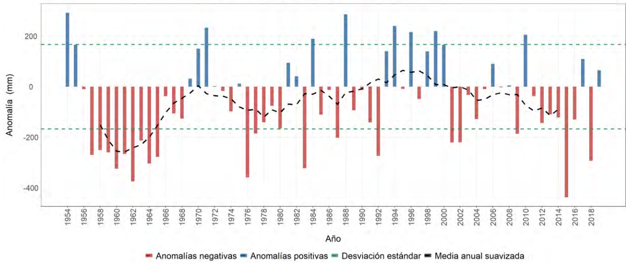
Estación meteorológica 5311503 - JULIO FERNÁNDEZ, Restrepo, Valle del Cauca Evolución anual de la anomalía de precipitación Promedio del periodo base (1981-2010): 1148 mm
