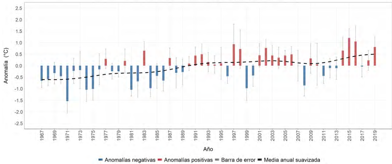
Estación meteorológica 2620502 - EL ROSARIO, Venecia, Antioquia Evolución anual de la anomalía de temperatura máxima media Promedio del periodo base (1981-2010): 25 °C
