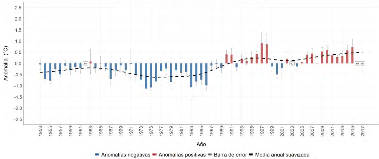
Estación meteorológica 5205507 - OSPINA PÉREZ, Consacá, Nariño Evolución anual de la anomalía de temperatura mínima media Promedio del período base (1981-2010): 15.3 °C
