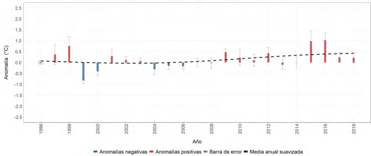
Estación meteorológica 5203503 - EL SAUCE, La Unión, Nariño Evolución anual de la anomalía de temperatura mínima media Promedio del período base (1981-2010): 16.1 °C
