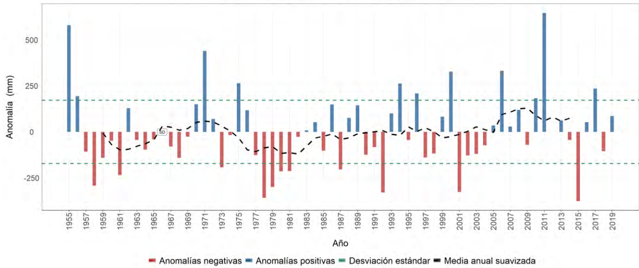
Estación meteorológica 2106503 - JORGE VILLAMIL, Gigante, Huila Evolución anual de la anomalía de precipitación Promedio del periodo base (1981-2010): 1340 mm
