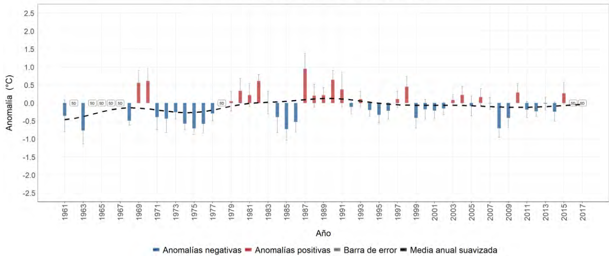
Estación meteorológica 2613507 - EL CEDRAL, Pereira, Risaralda Evolución anual de la anomalía de temperatura mínima media Promedio del periodo base (1981-2010): 11.4 °C
