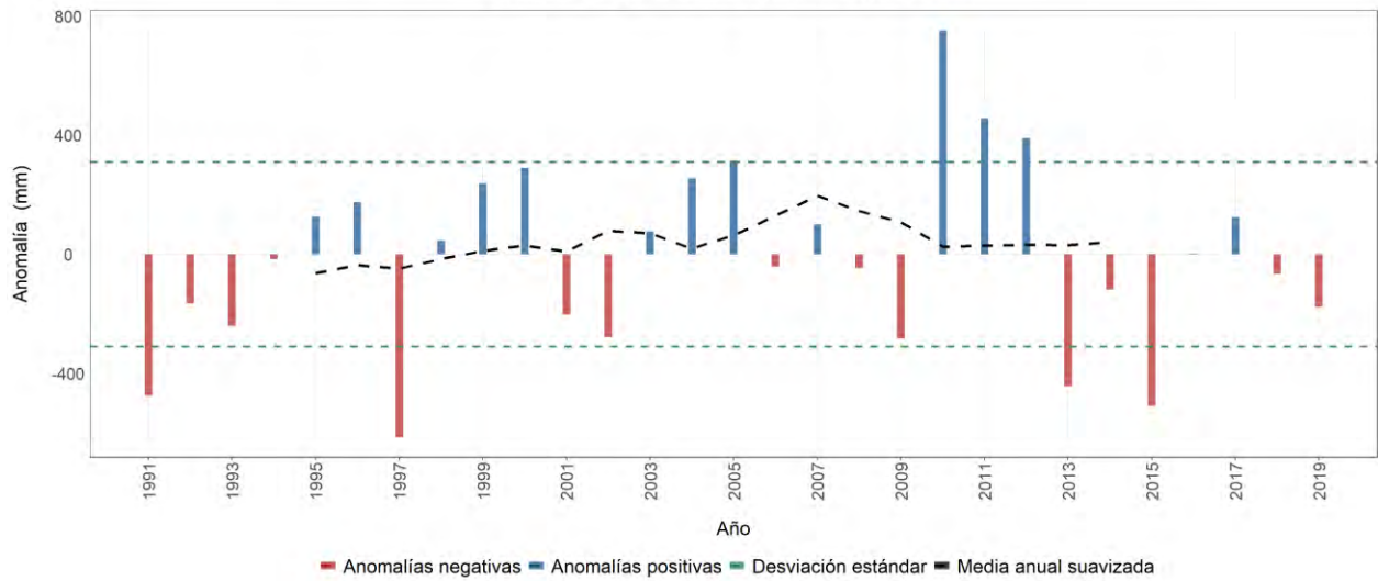
Estación meteorológica 1605511 - GABRIEL MARÍA BARRIGA, Convención, Norte de Santander Evolución anual de la anomalía de precipitación Promedio del periodo base (1981-2010): 1190 mm
