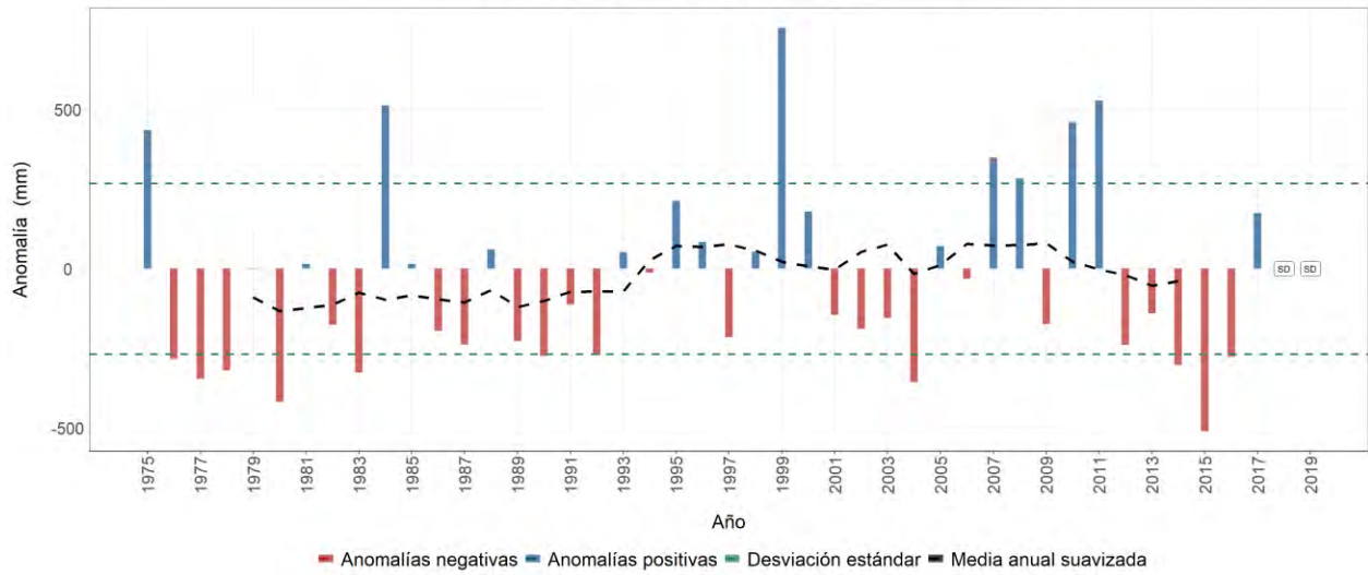
Estación meteorológica 5403503 - ALBÁN, El Cairo, Valle del Cauca Evolución anual de la anomalía de precipitación Promedio del periodo base (1981-2010): 1531 mm
