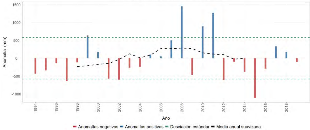
Estación meteorológica 2614026 - LA ELVIRA, Belén De Umbría, Risaralda Evolución anual de la anomalía de precipitación Promedio del período base (1981-2010): 2404 mm
