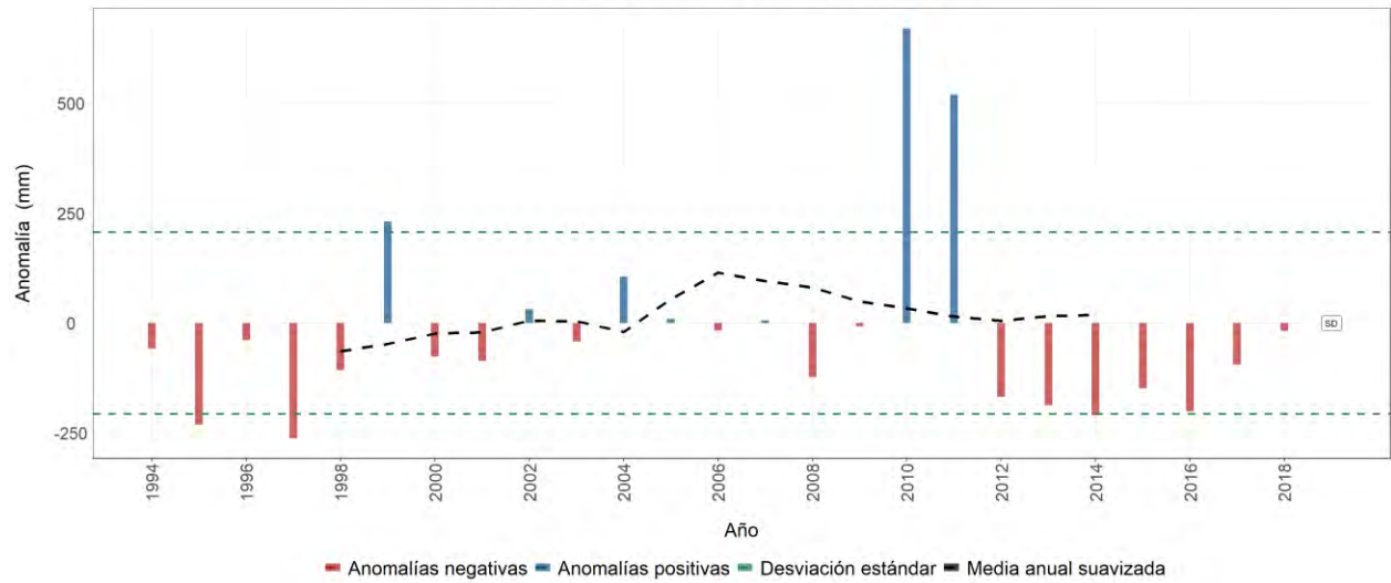
Estación meteorológica 741 - ALBERTO SANTOS, Socorro, Santander Evolución anual de la anomalía de precipitación Promedio del periodo base (1981-2010): 1619 mm
