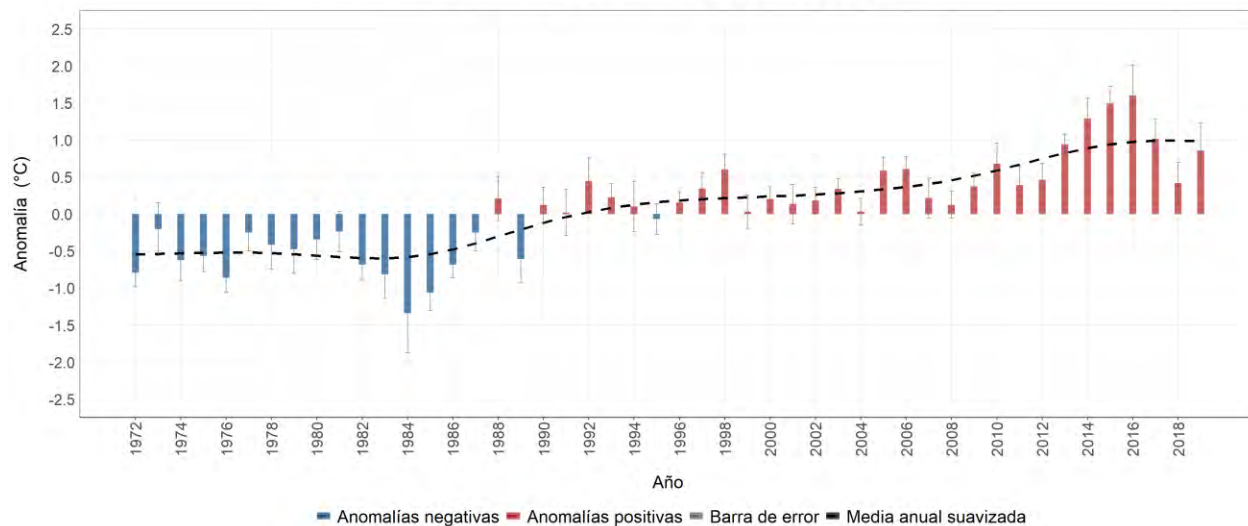
Estación meteorológica 2615514 - GRANJA LUKER, Palestina, Caldas Evolución anual de la anomalía de temperatura mínima media Promedio del período base (1981-2010): 18.1 °C
