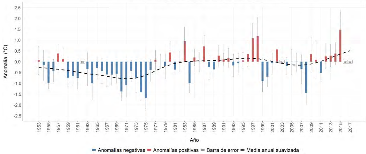
Estación meteorológica 5205507 - OSPINA PÉREZ, Consacá, Nariño Evolución anual de la anomalía de temperatura máxima media Promedio del período base (1981-2010): 25.2 °C
