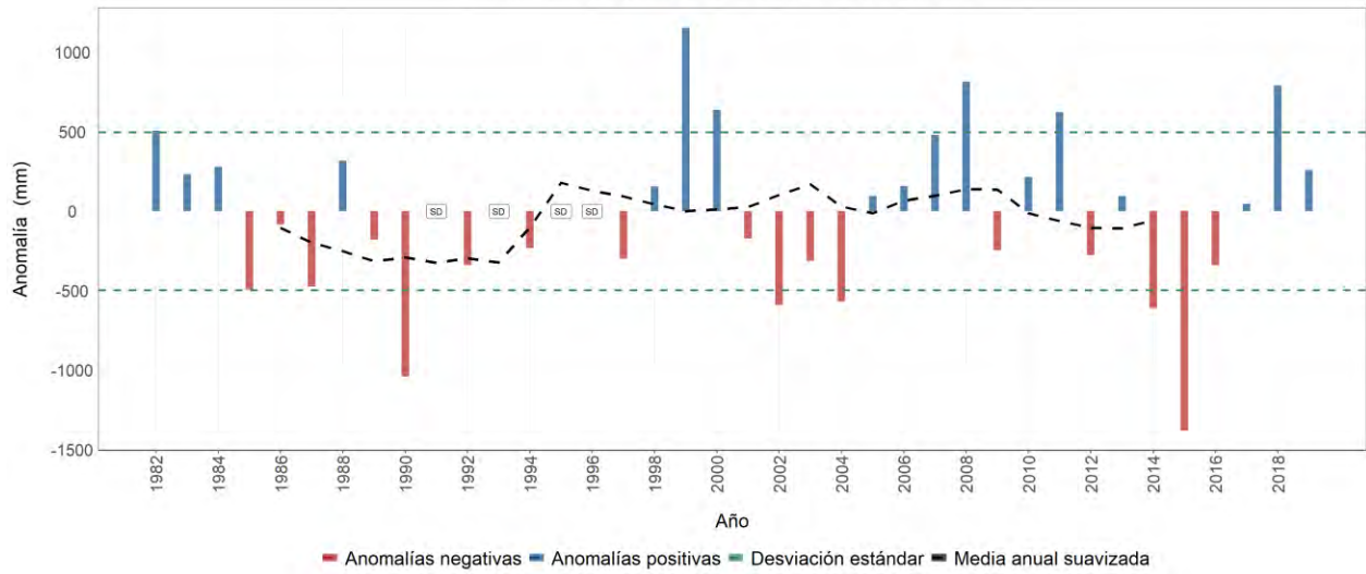
Estación meteorológica 2612021 - LA ILUSIÓN, Circasia, Quindío Evolución anual de la anomalía de precipitación Promedio del período base (1981-2010): 2579 mm
