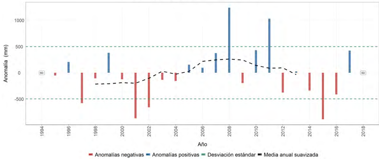
Estación meteorológica 6 - LA JULIANA, Manizales, Caldas Evolución anual de la anomalía de precipitación Promedio del período base (1981-2010): 2083 mm
