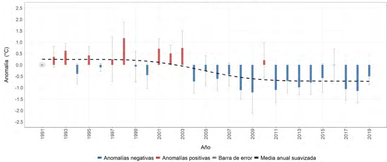
Estación meteorológica 1605511 - GABRIEL MARÍA BARRIGA, Convención, Norte de Santander Evolución anual de la anomalía de temperatura máxima media Promedio del período base (1981-2010): 25.4 °C
