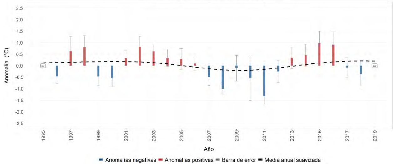
Estación meteorológica 741 - ALBERTO SANTOS, Socorro, Santander Evolución anual de la anomalía de temperatura máxima media Promedio del período base (1981-2010): 26.7 °C
