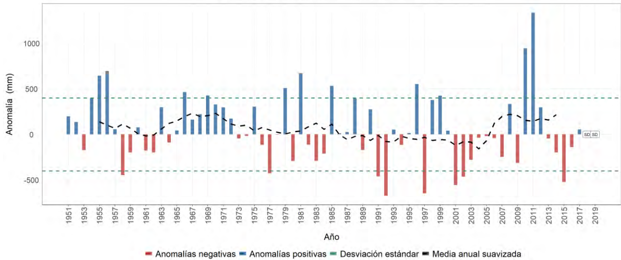
Estación meteorológica 1601506 - BLONAY, Chinácota, Norte de Santander Evolución anual de la anomalía de precipitación Promedio del periodo base (1981-2010): 1406 mm
