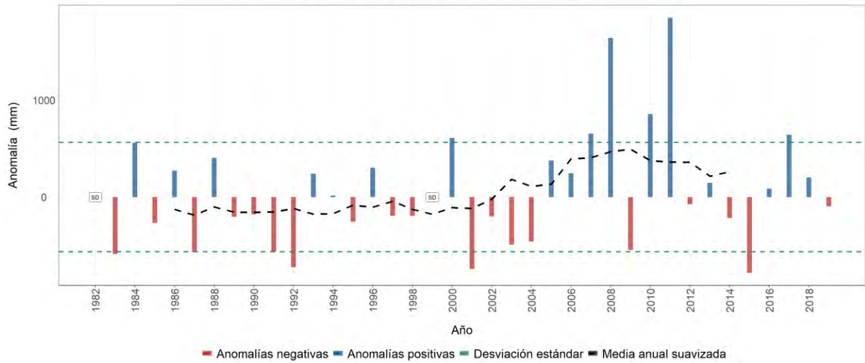
Estación meteorológica 2612059 - LA ESPERANZA, Buenavista, Quindío Evolución anual de la anomalía de precipitación Promedio del periodo base (1981-2010): 2324 mm
