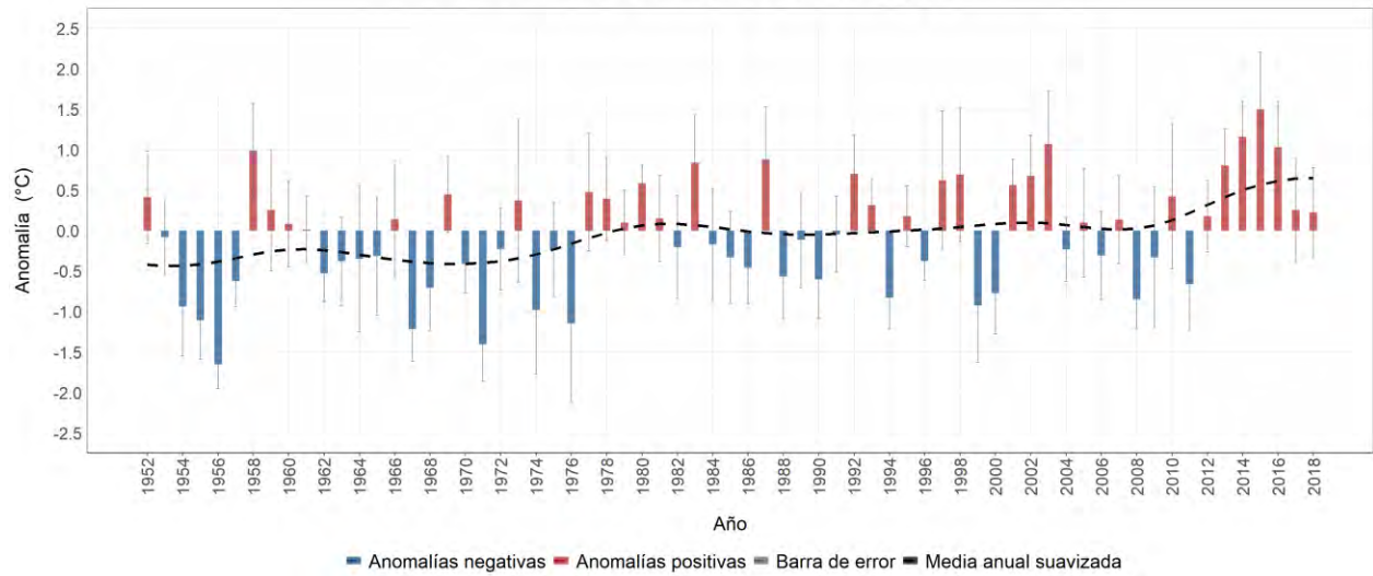
Estación meteorológica 1601506 - BLONAY, Chinácota, Norte de Santander Evolución anual de la anomalía de temperatura máxima media Promedio del período base (1981-2010): 26.2 °C
