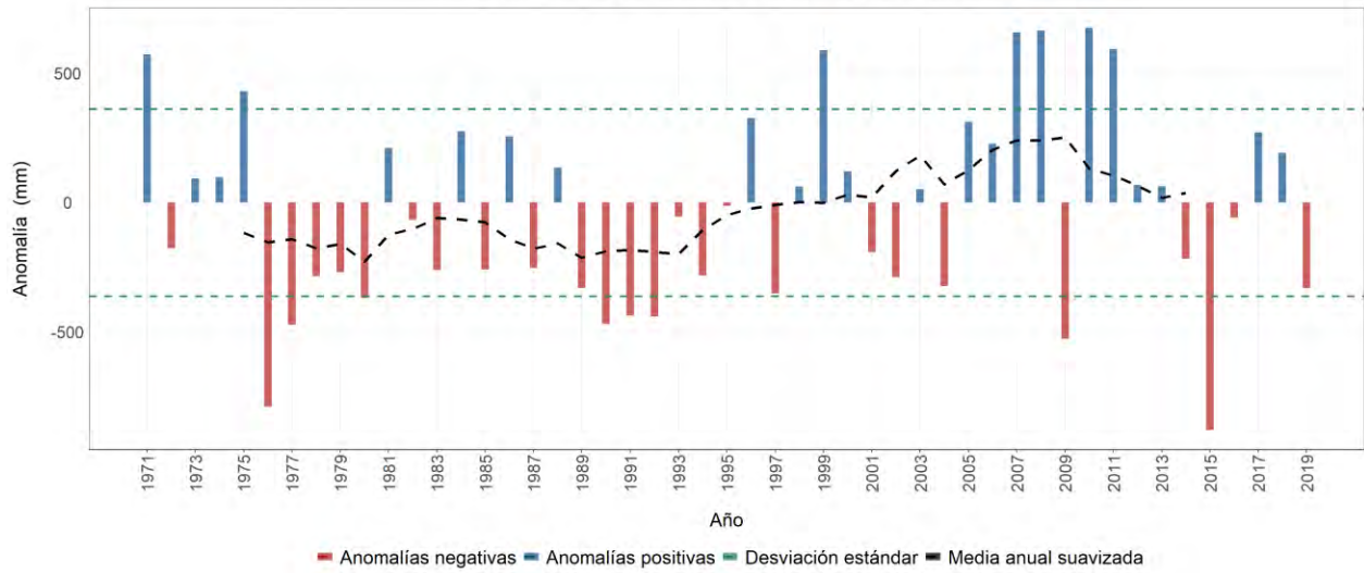
Estación meteorológica 2617507 - RAFAEL ESCOBAR, Supía, Caldas Evolución anual de la anomalía de precipitación Promedio del período base (1981-2010): 2034 mm
