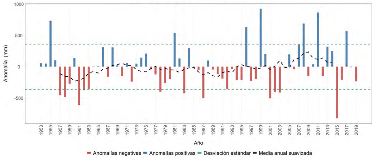
Estación meteorológica 2603506 - MANUEL MEJÍA, El Tambo, Cauca Evolución anual de la anomalía de precipitación Promedio del período base (1981-2010): 2060 mm
