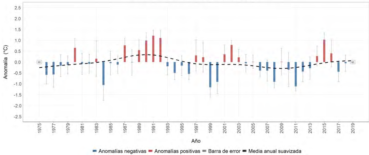
Estación meteorológica 2613506 - EL JAZMÍN, Santa Rosa De Cabal, Risaralda Evolución anual de la anomalía de temperatura máxima media Promedio del período base (1981-2010): 24.6 °C
