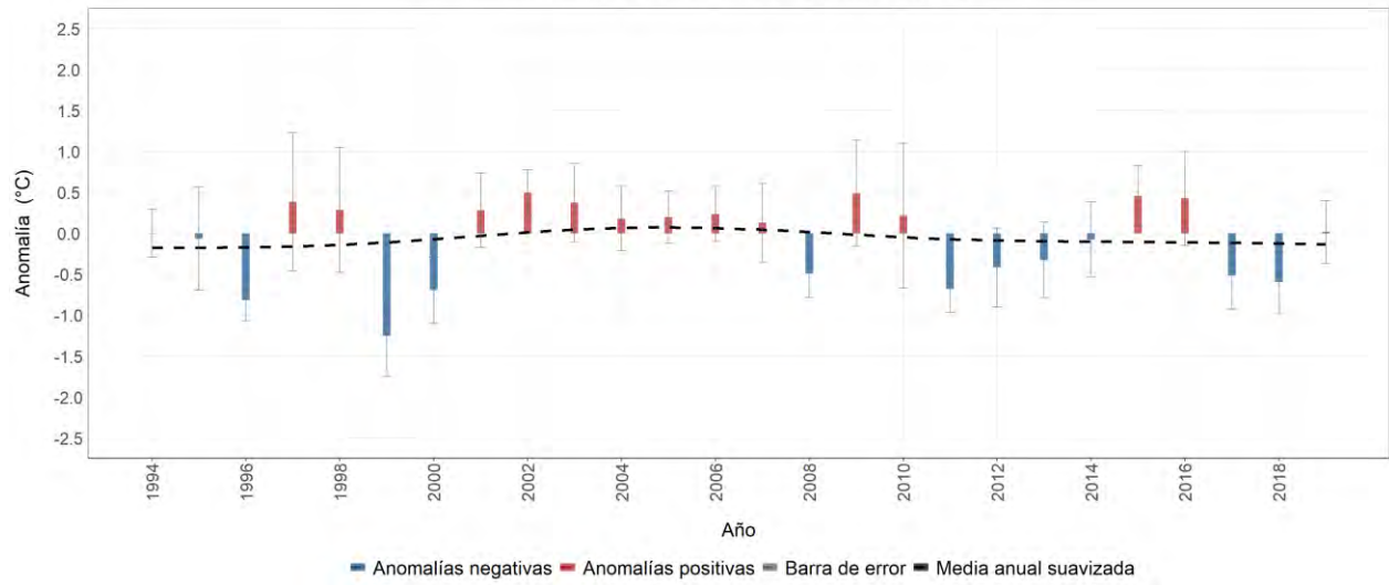
Estación meteorológica 37 - PLANALTO, Manizales, Caldas Evolución anual de la anomalía de temperatura máxima media Promedio del período base (1981-2010): 26.6 °C
