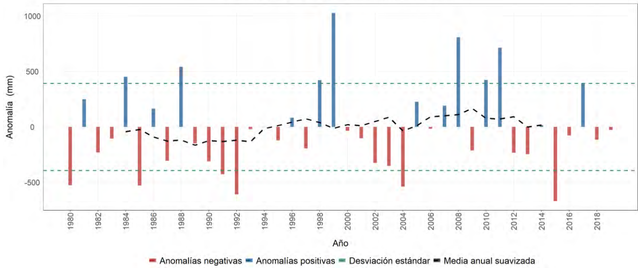
Estación meteorológica 2612523 - EL AGRADO, Montenegro, Quindío Evolución anual de la anomalía de precipitación Promedio del período base (1981-2010): 2134 mm
