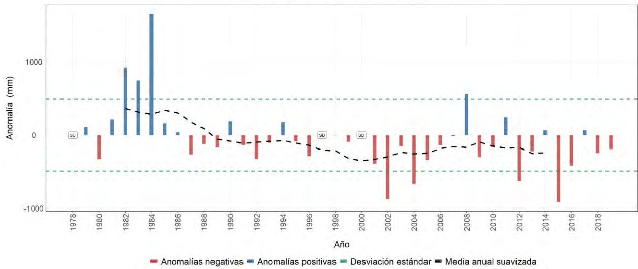
Estación meteorológica 2602041 - LA TRINIDAD, Piendamó, Cauca Evolución anual de la anomalía de precipitación Promedio del período base (1981-2010): 2292 mm
