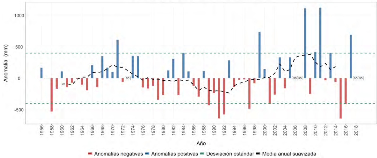
Estación meteorológica 2615505 - AGRONOMÍA, Manizales, Caldas Evolución anual de la anomalía de precipitación Promedio del periodo base (1981-2010): 1893 mm
