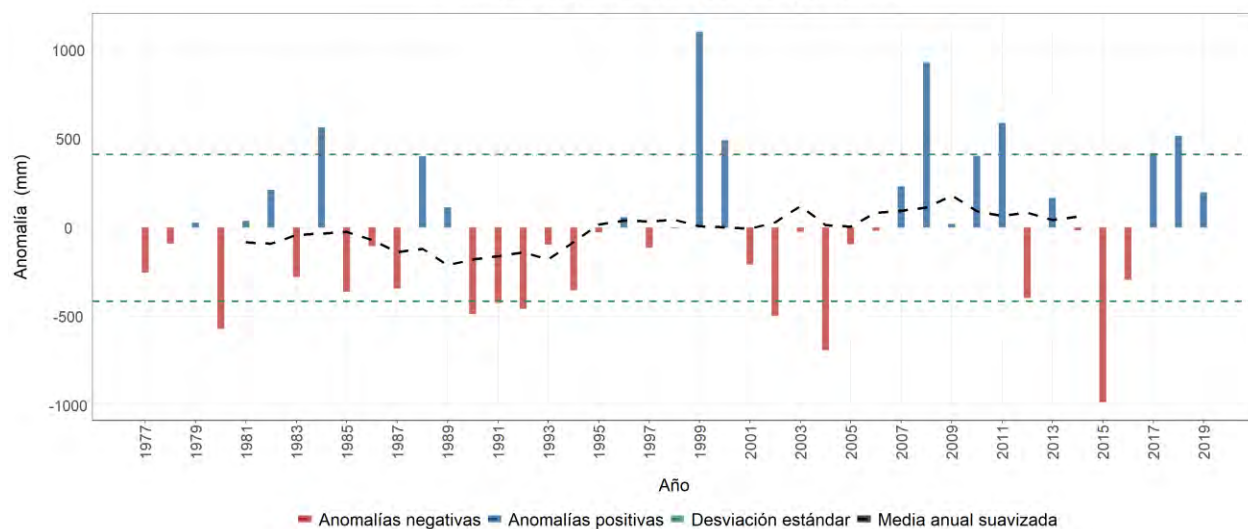
Estación meteorológica 2612525 - MARACAY, Quimbaya, Quindío Evolución anual de la anomalía de precipitación Promedio del período base (1981-2010): 2462 mm
