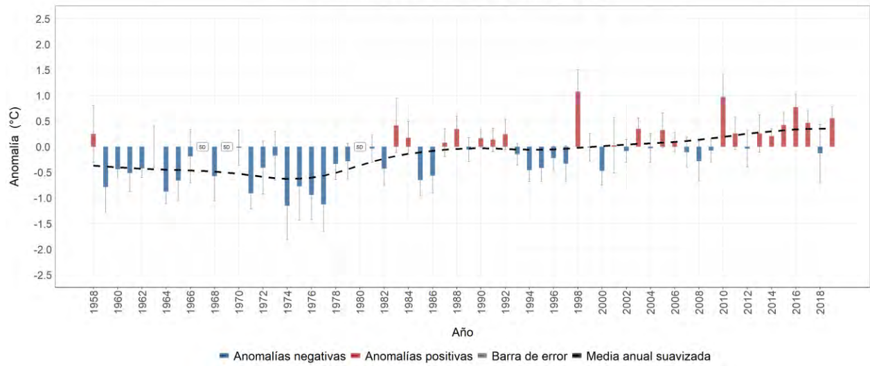
Estación meteorológica 2804501 - PUEBLO BELLO, Valledupar, Cesar Evolución anual de la anomalía de temperatura mínima media Promedio del período base (1981-2010): 15.8 °C
