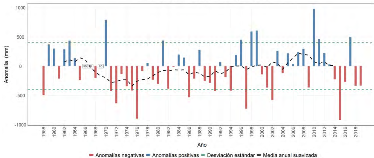
Estación meteorológica 2804501 - PUEBLO BELLO, Valledupar, Cesar Evolución anual de la anomalía de precipitación Promedio del período base (1981-2010): 2059 mm
