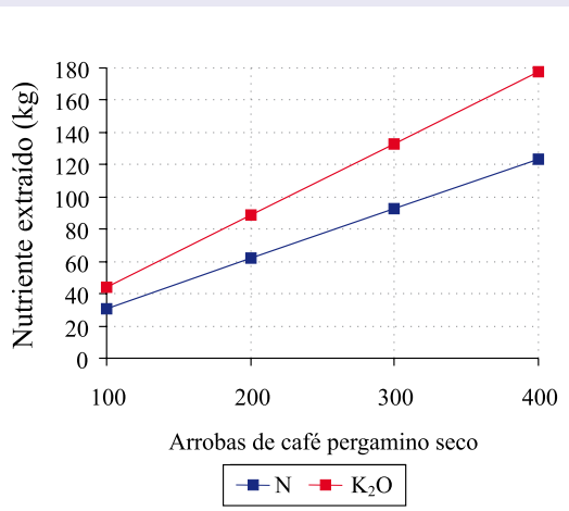
Figura 4. Cantidades de nitrógeno (N) y potasio ( K_2O ) extraídas por cosechas de 100 a 400 arrobas de c.p.s.
