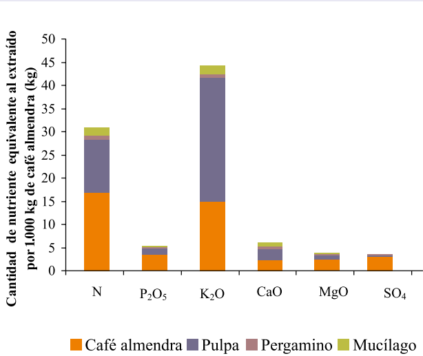
Figura 2. Extracción de macronutrientes por las partes que componen el fruto del café de la variedad Colombia.
