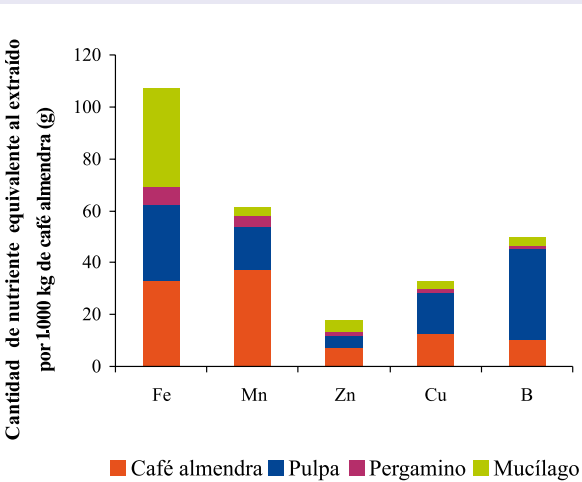
Figura 3. Extracción de micronutrientes por las partes que componen el fruto del café de la variedad Colombia.
