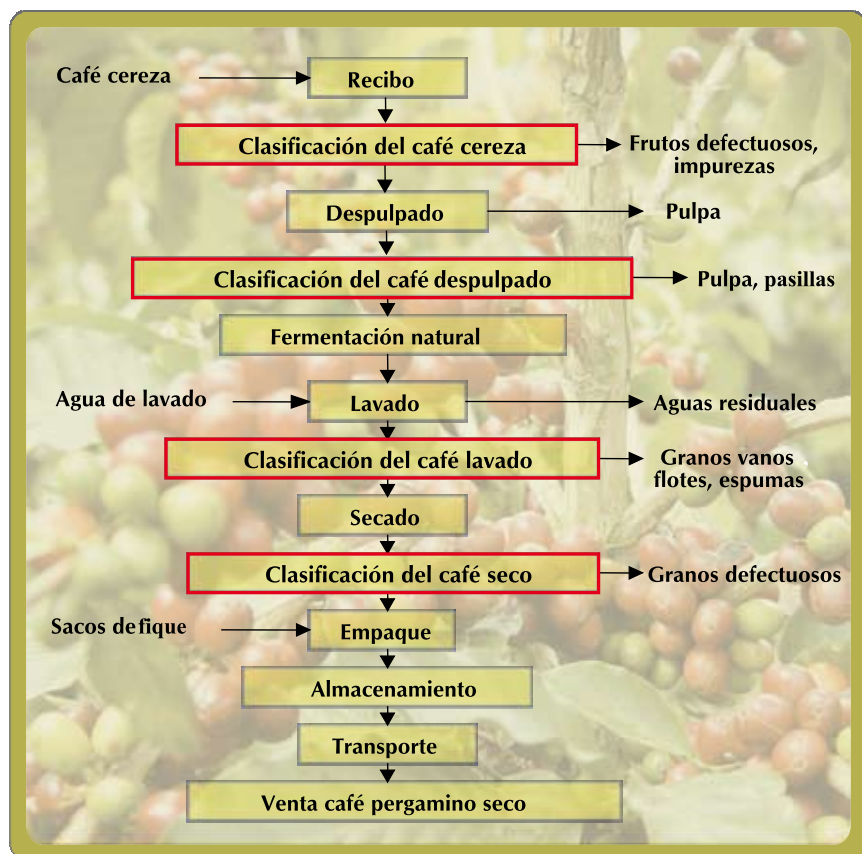
Figura 3. Flujo del proceso controlado de beneficio del café.
