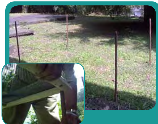
Figura 4. Base en madera macana para piso en tierra
