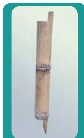
Figura 3. Base de guadua para piso en tierra. Corte en estaca y patilla.
