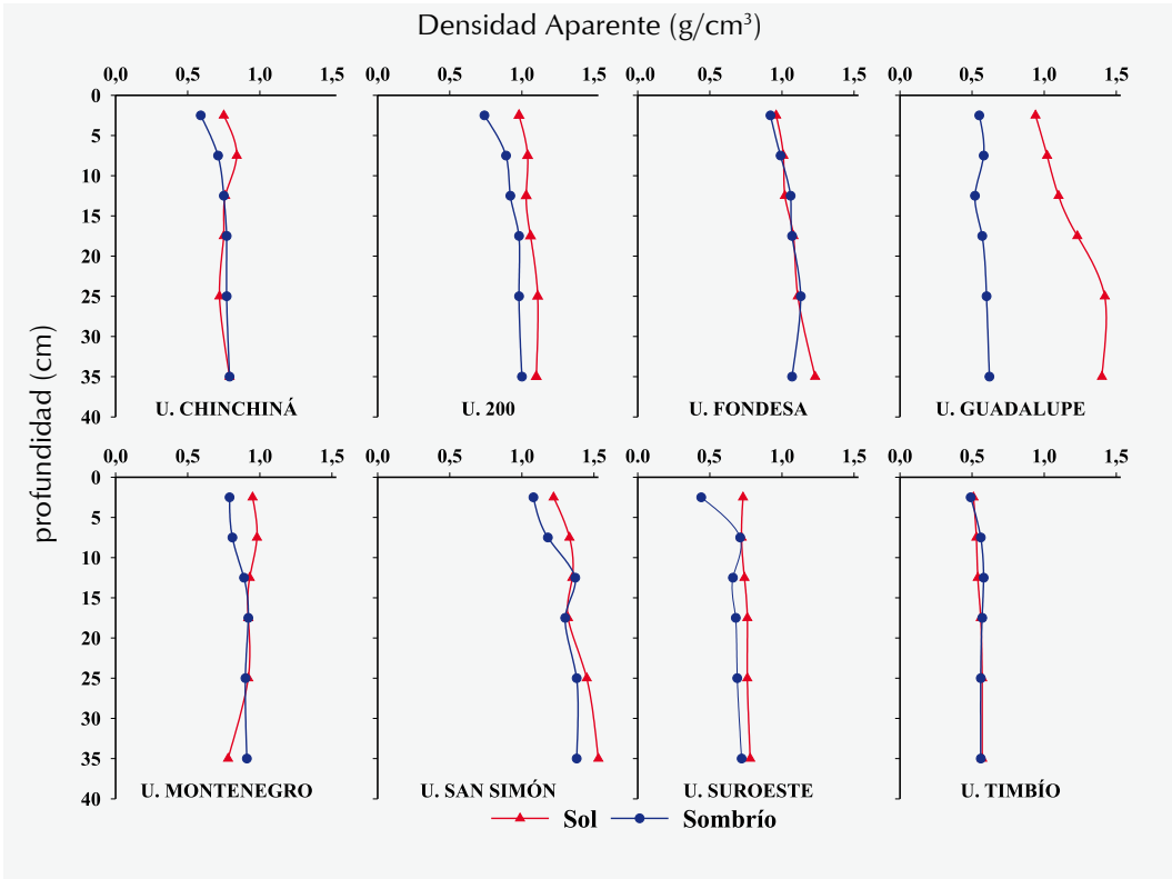
Figura 2. Tendencia de la densidad aparente (g/cm 3 ) a diferentes profundidades, en las ocho unidades de suelo evaluadas en la zona cafetera colombiana.
