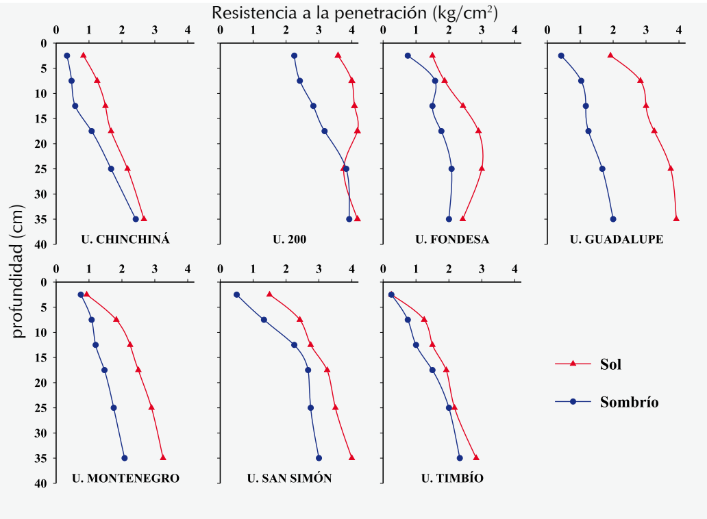
Figura 4. Tendencia de la resistencia a la penetración (kg/cm²) a diferentes profundidades, en siete unidades de suelo evaluadas en la zona cafetera colombiana.
