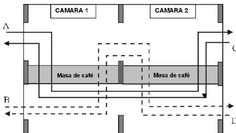
Figura 5. Esquema de un silo-secador “Cenicafé”
