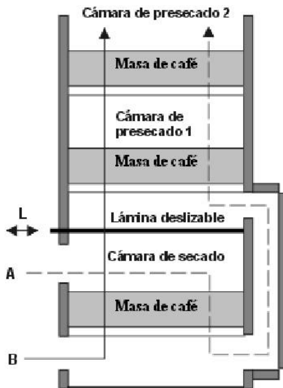
Figura 9. Esquema de un secador de tres pisos
