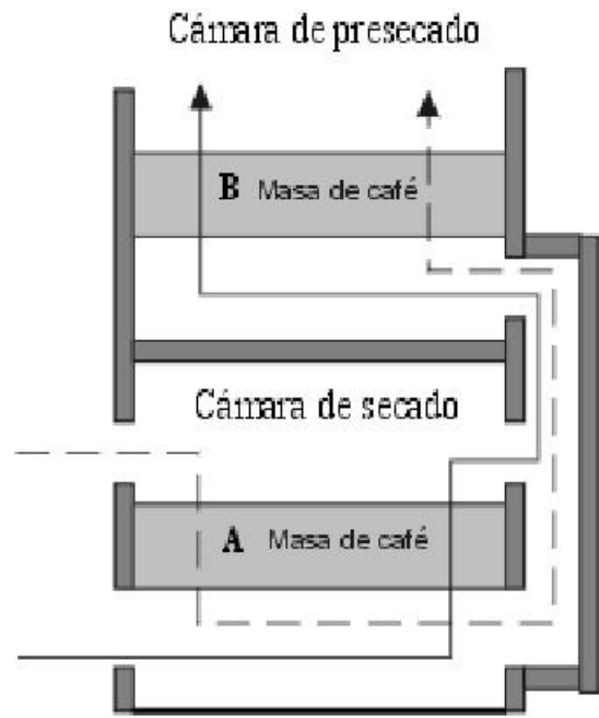
Figura 7. Esquema de un secador de café de dos pisos (Silo-secador Vertical) y la manera como opera
