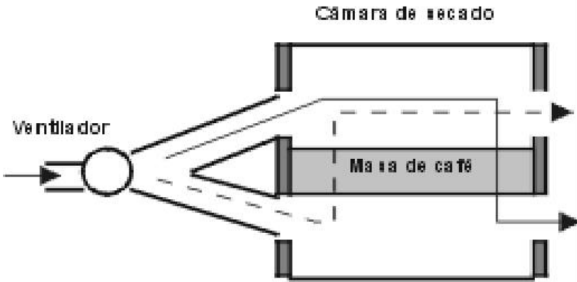
Figura 3. Esquema de un secador estacionario de café sin cámara de presecado y con inversión del flujo de aire.
