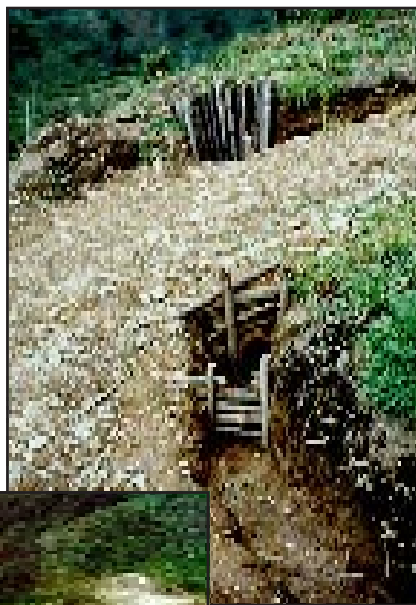
Figura 10. Caja colectora de aguas de escorrentía.
