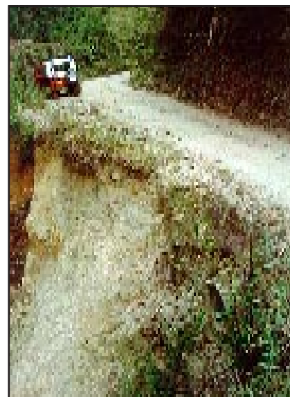
Figura 8. Formación de negativo de carretera por obras inconclusas
