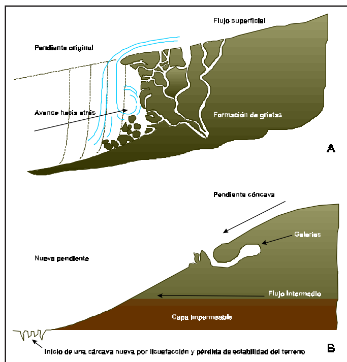
Figura 3. Dibujo que representa el proceso mediante el cual se amplía una cárcava. En la medida que la cabeza de la cárcava retrocede, es mayor la altura de caída del agua; el efecto de cascada erosiona el suelo, ya que salpica y arremolina contra el escarpe, dejando la parte alta en saliente.
