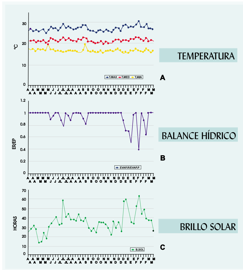
Figura 6. Condiciones climáticas durante el período marzo del 94 a marzo del 95. A. Temperatura (°C). B. Balance hídrico (evaporación potencial/evaporación real. C. Brillo solar (Horas)
