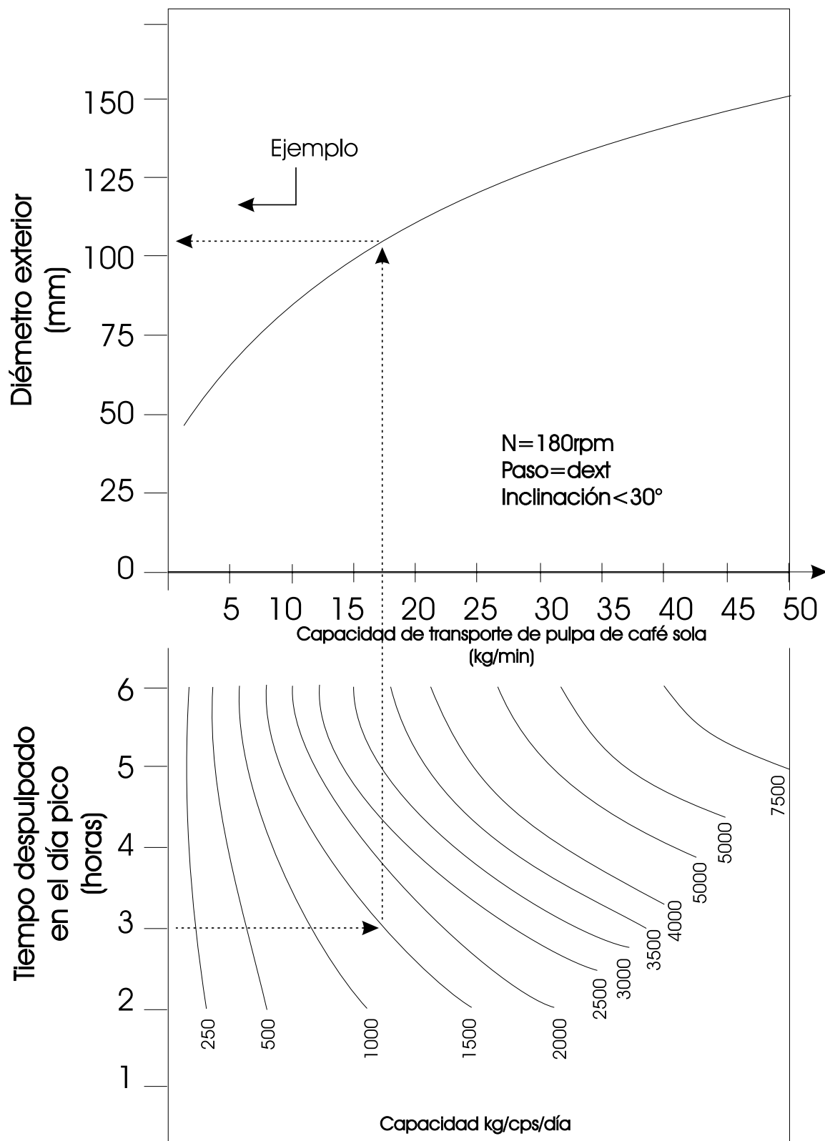
Figura 4. Curvas para la selección del diámetro exterior en transportadores de tornillo sinfín para pulpa de café sola o mezclada con mucílago concentrado
