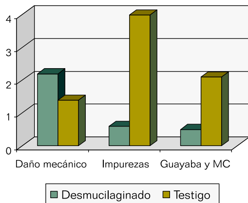
Figura8. Daño mecánico, Impurezas y Guayabas y Mdia Cara (MC) obtenidos en el desmucilaginador CENICAFÉ El Granjero y con el beneficio tradicional (testigo).
