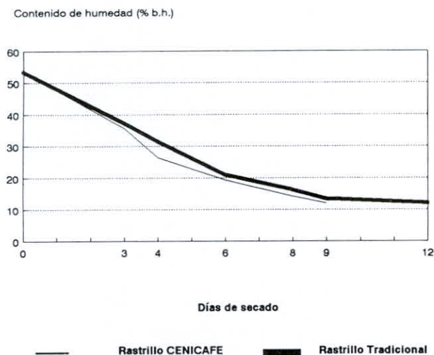
Figura 6. Relación entre el tiempo de secado y su contenido de humedad.
