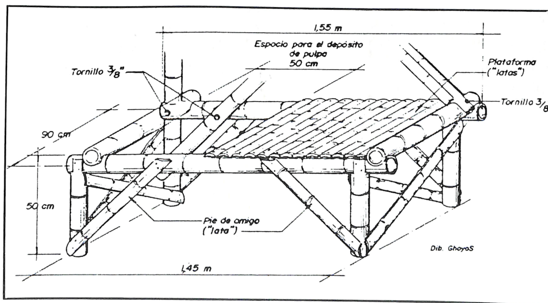
Figura 3. Plataforma y bastider.
