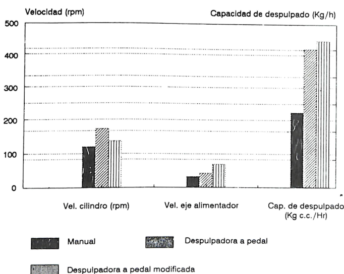
Figura 8. Desempeño comparativo de la despulpadora a pedal.
