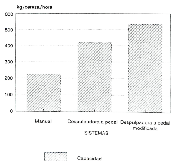
Figura 9. Evaluación de la despulpadora a pedal modificada.
