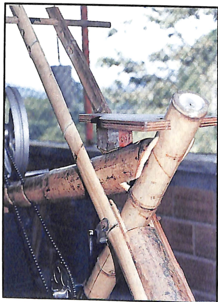
Detalle A. Ensamble del marco de guadua, el sillín y el manubrio.
