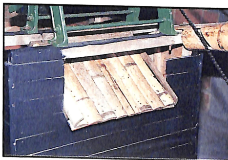
Detalle B. Tobogán para el descargo de la pulpa.
