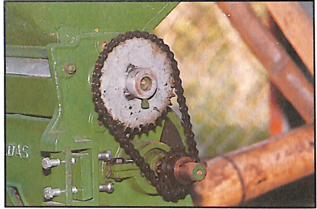
Figura 4. Modificación de la velocidad angular del eje alimentador mediante el cambio de la relación de piñones.
