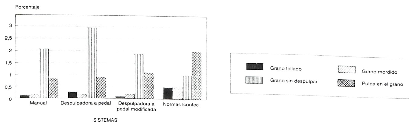
Figura 10. Despulpadora de café a pedal. Análisis de calidad de despulpado.
