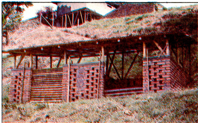
Figura 5. Fosas de ladrillo de fácil construcción. Nótase el aprovechamiento de la pendiente para el arrastre de la pulpa.
