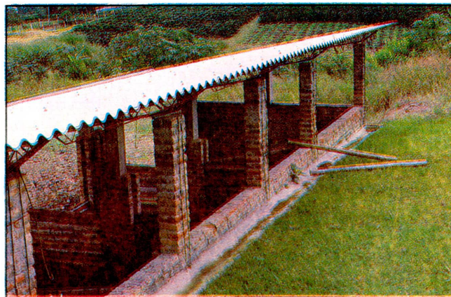
Figura 6. Escurridero para evitar que el agua entre a la fosa.
