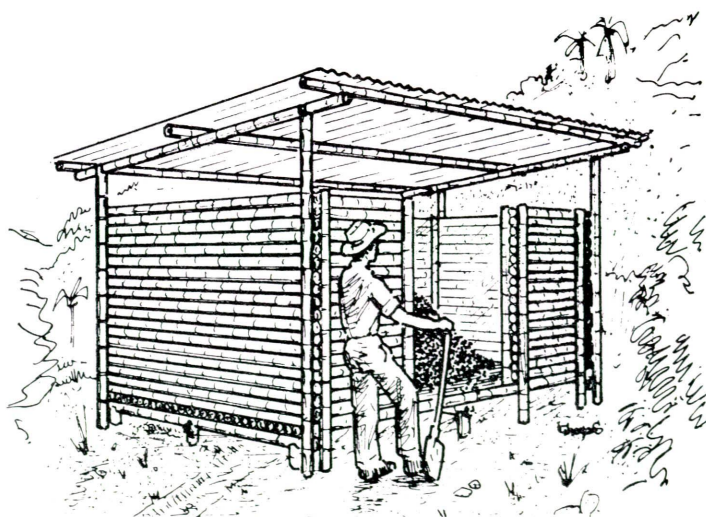
Figura 4. Chiquero de guadua para descomposición de la pulpa. Apropiado para pequeños productores.
