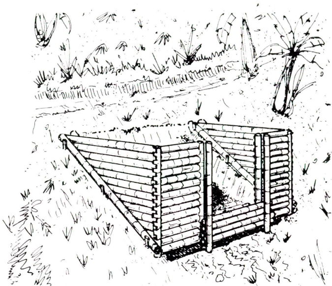
Figura 3. Fosa en tierra complementada con guadua.
