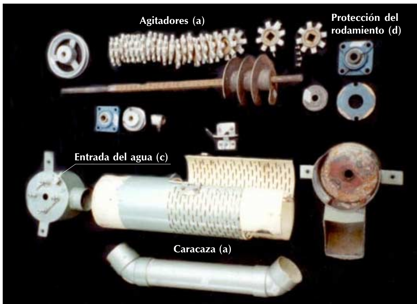
Figura 2. Detalles del DESLIM 300. Carcaza (a), agitadores (b), suministro de agua (c) y protección del rodamiento inferior(d).
