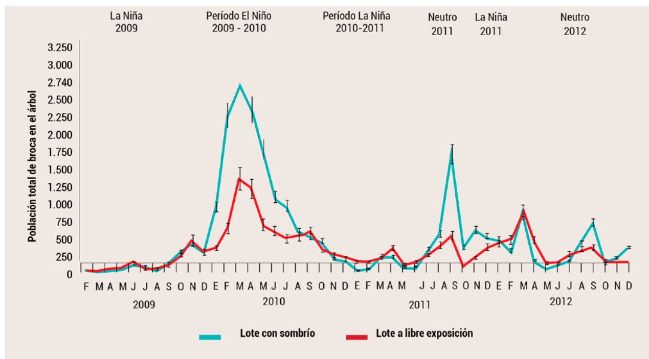
Figura 3. . Cambios en la densidad poblacional de broca por árbol en sistemas de producción con café a libre exposición solar y bajo sombra durante cuatro cosechas al año para un ciclo productivo de cinco años en Naranjal (Chinchiná-Caldas), en diferentes fases ENOS “La Niña”, “El Niño” y “Neutro” (Constantino et al., 2021).
