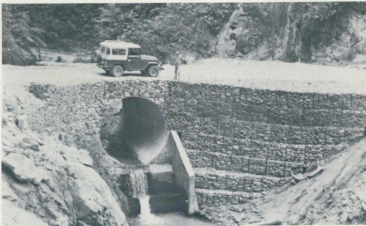
Alcantarilla con gaviones. Quebrada Ondas. Vía Ríoblanco - Santafé.
