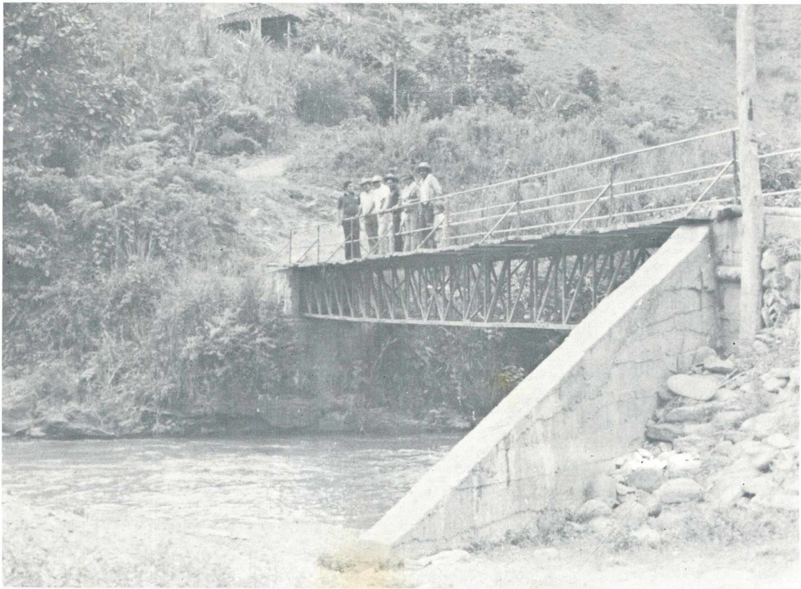
Puente Peatonal El Sinai Luz Libre: 22 mts. - Municipio Argelia.
