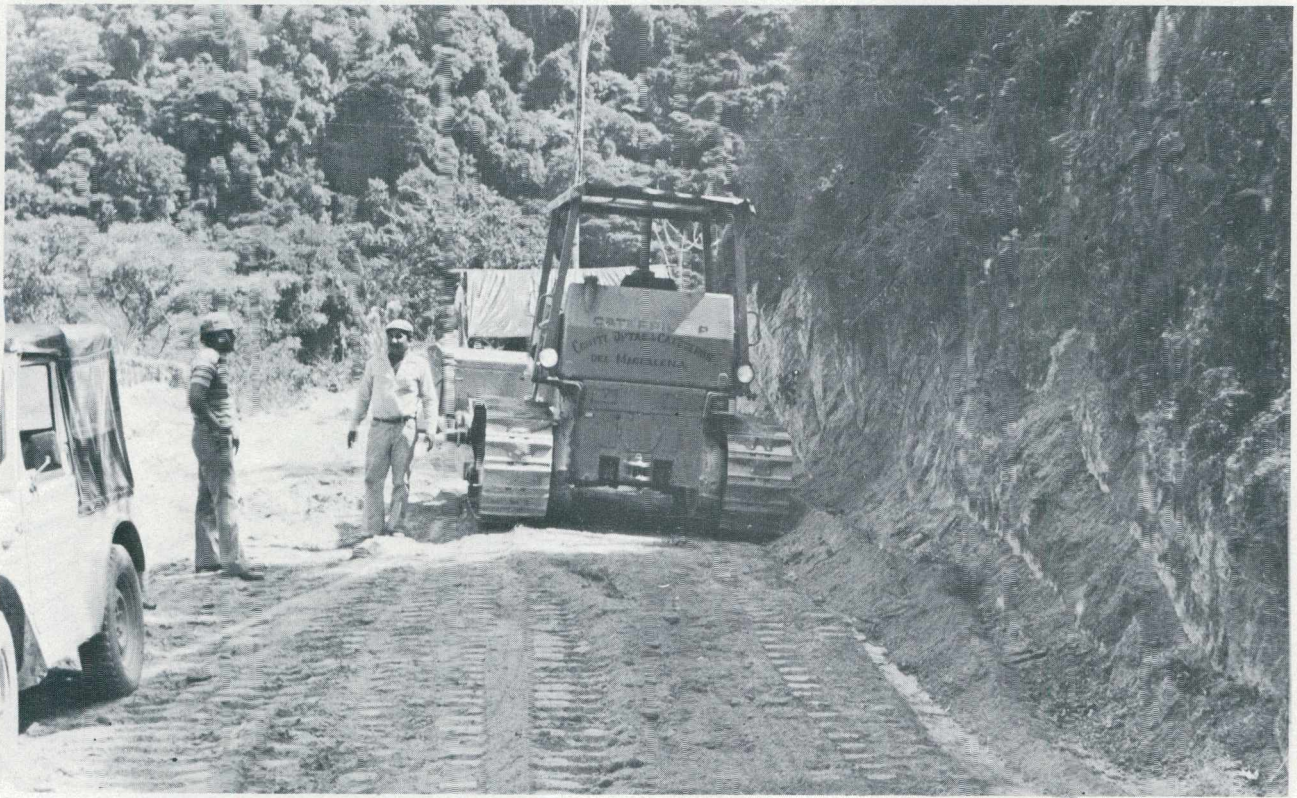
Construcción tramo carretable Minca - Las Minas
