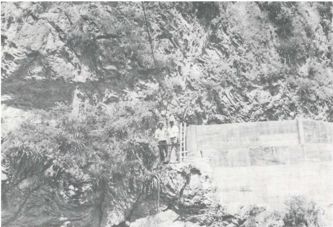
Estribo para puente sobre el río Guaitará, Vía Sotomayor-Río Guaitará - Peñol.
