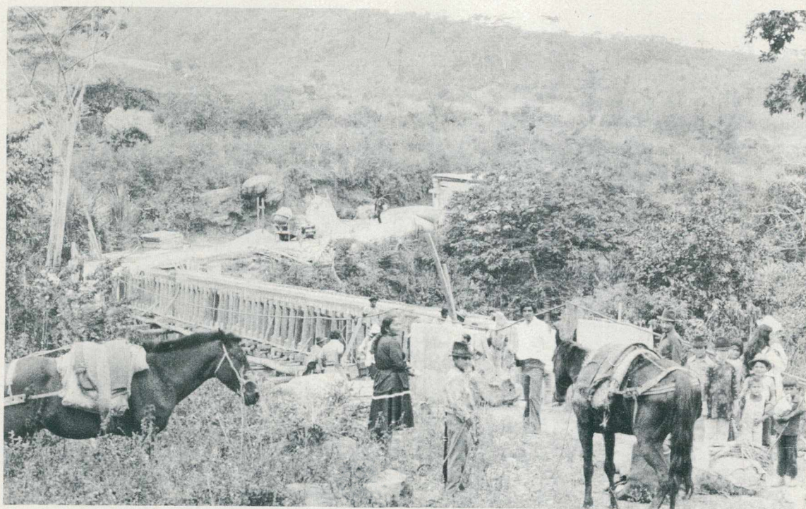
Puente sobre el Río Ubaza, Municipio San José de Pare, Luz 28 metros.
