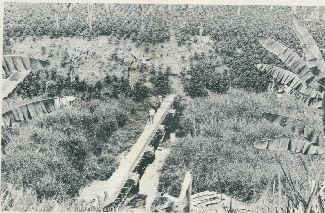
Viaducto sobre quebrada Cristales. Acueducto Alto El Oso. Municipios Armenia, La Tebaida.
