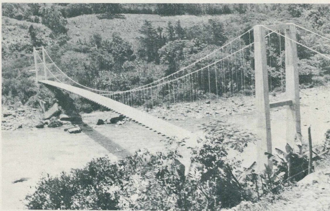
Puente peatonal Támara sobre el río Margua. Luz: 100 metros. Corregimiento San Berrardo. Municipio Toledo.
