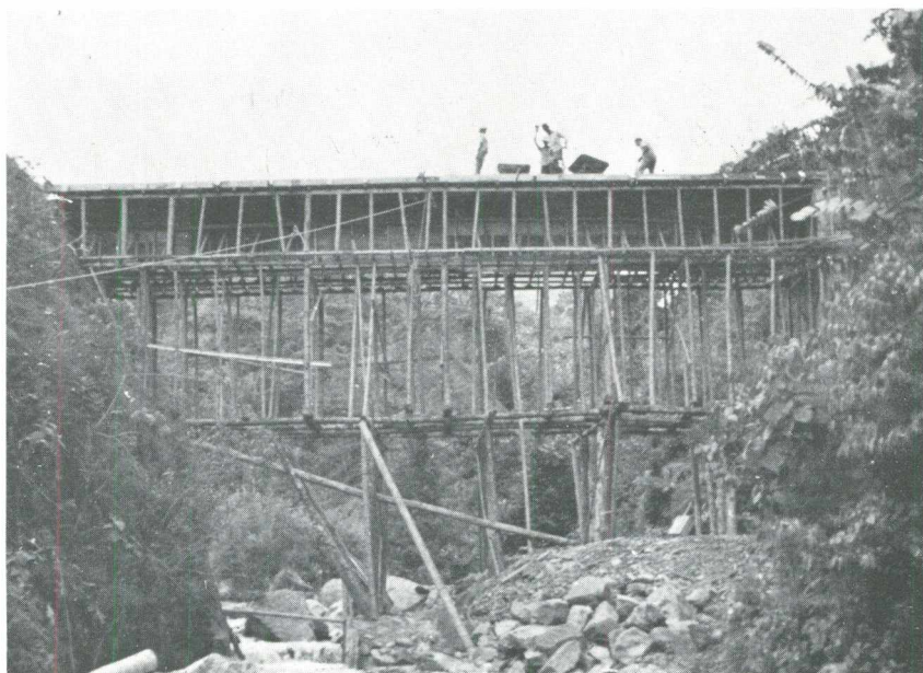
Puente peatonal La Maizena. Municipio: Pijao.
