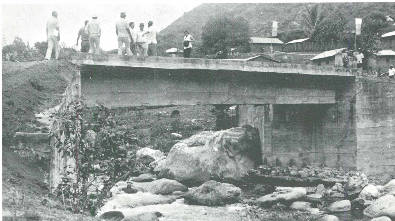
Puente Chemesquemena. Municipio: Valledupar. Luz: 16 mts.
