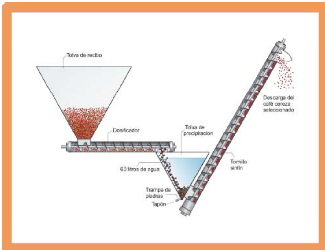
Figura 7. Esquema del separador hidráulico de tolva y tornillo sinfín desarrollado en Cenicafé por Oliveros y Col. (2007).
