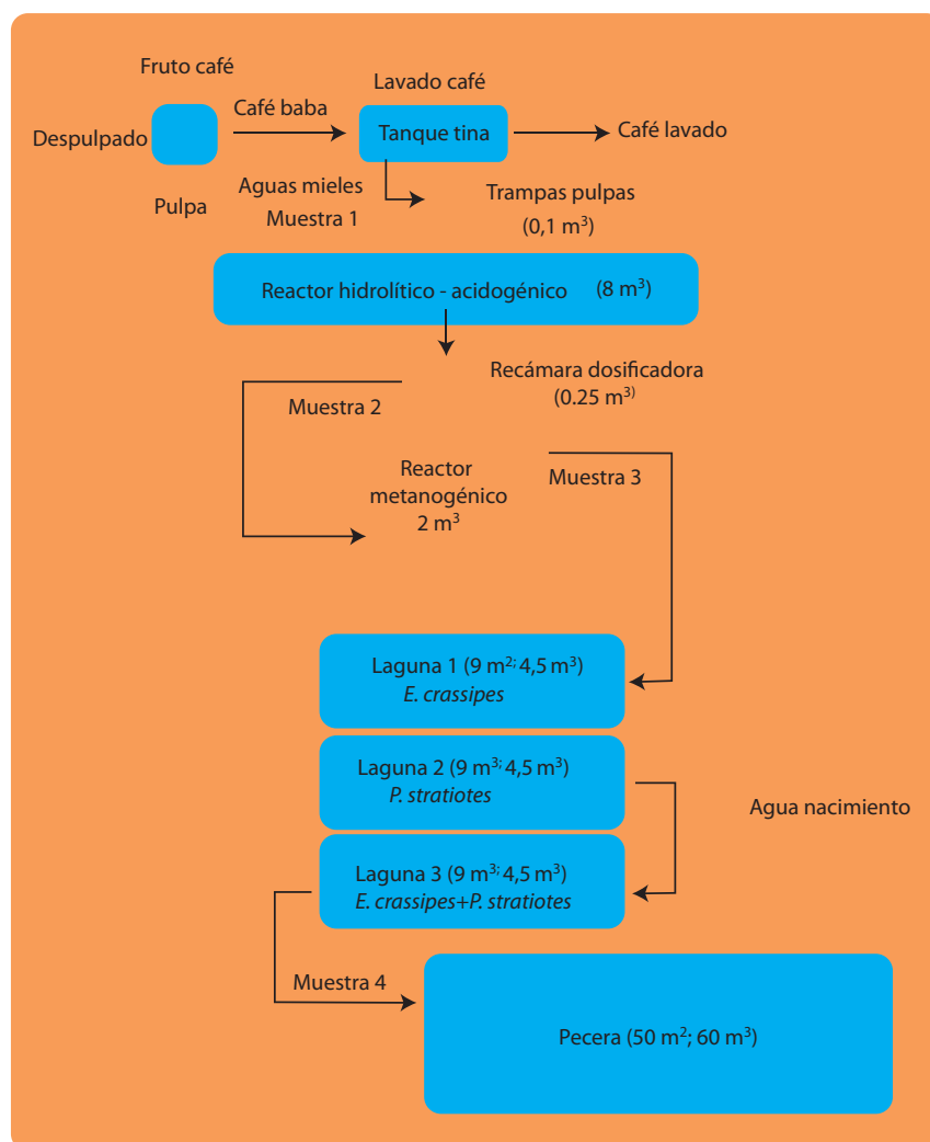
Figura 12. Esquema del sistema acuático de tratamiento acoplado al SMTA en una finca cafetera y localización de los puntos de muestreo.
