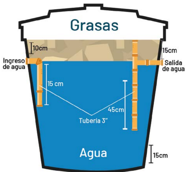
Figura 3. Esquema de una trampa de grasas construida en un tanque de polietileno de 250 L, con una altura útil de 0,75 m. Fuente: Adaptado de Rodríguez et al., 2018.
