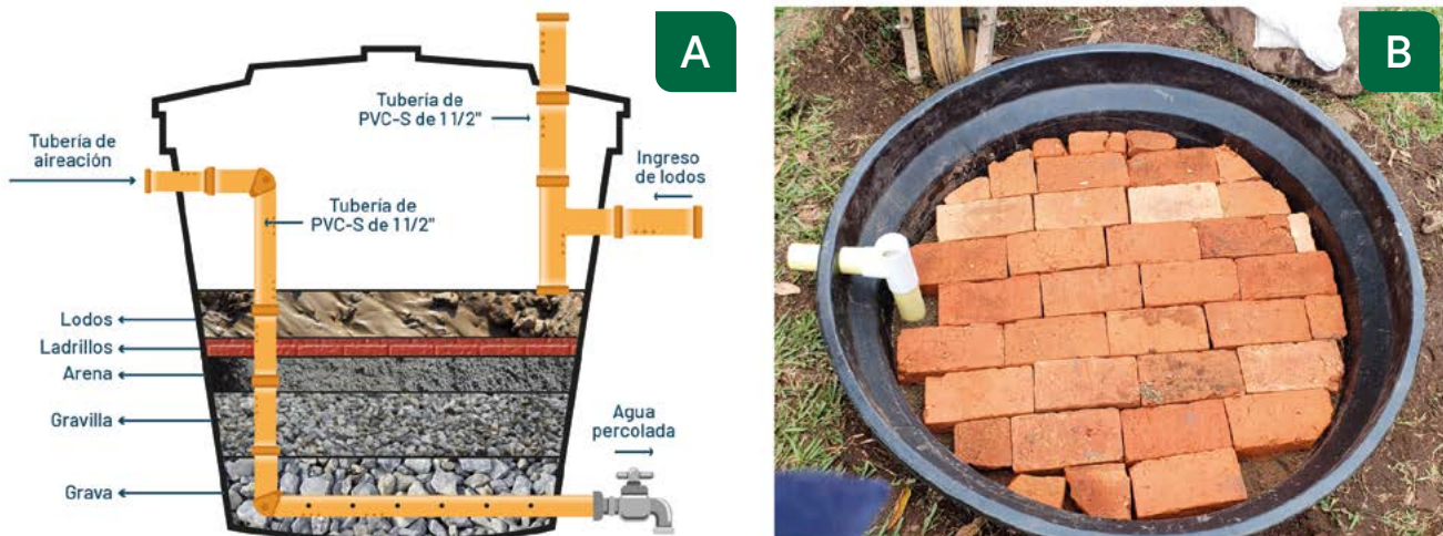
Figura 10. Tanque en polietileno adaptado como lecho de secado de lodos A. Esquema. B. Aspecto en el campo (Rodríguez et al., 2022b).
