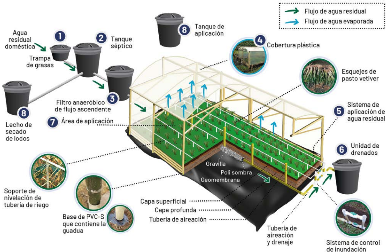
Figura 14. Aspecto de un sistema de manejo y tratamiento de las ARD-T incorporando un filtro verde con cero descargas.
