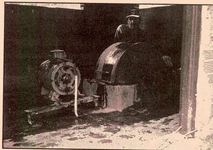
La rueda Pelton y el generador
