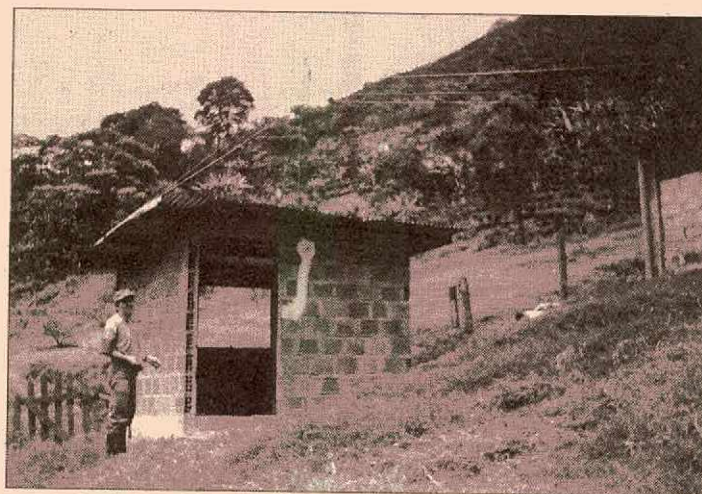
Caseta donde está instalada la rueda Pelton.
