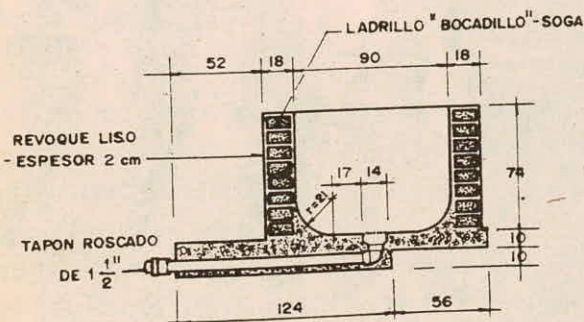
CORTE TRANSVERSAL
