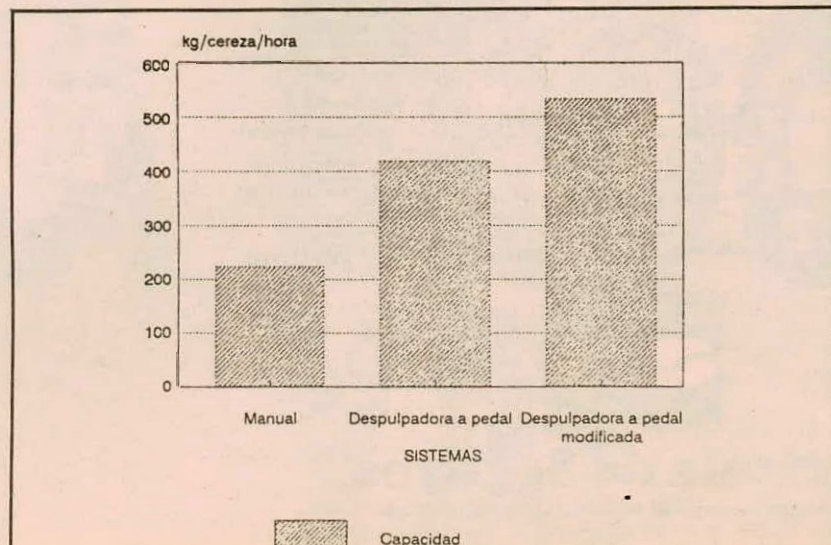
FIGURA 3. Evaluación de la despulpadora a pedal modificada.
