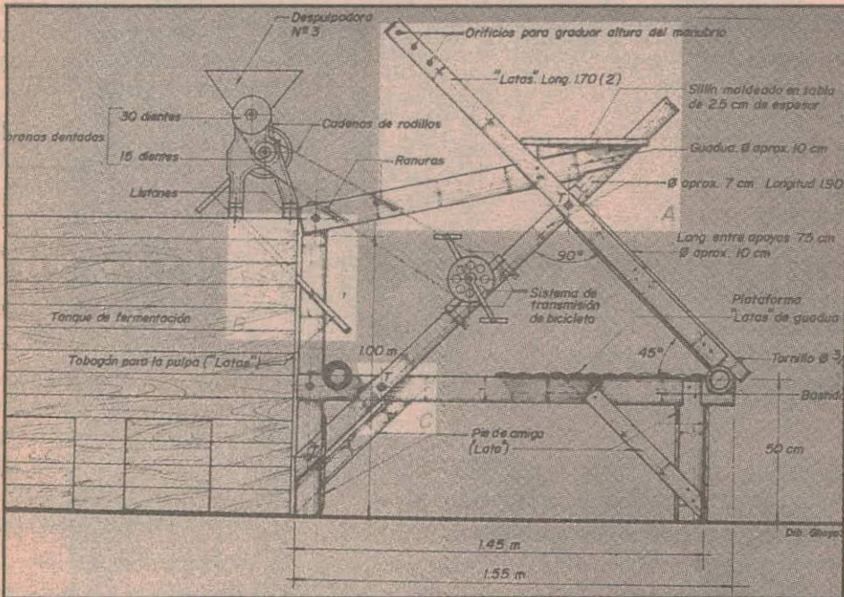
FIGURA 1. Vista lateral del sistema de despulpado y detalles de construcción de la estructura de pedaleo.
