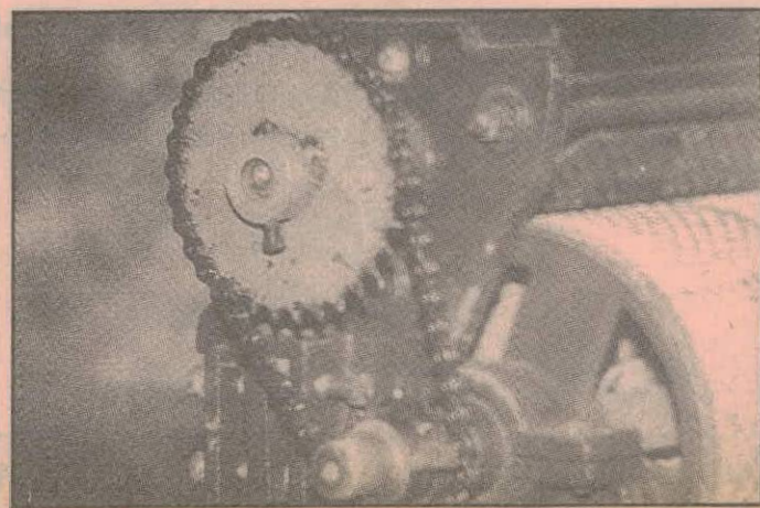
Modificación de la velocidad angular del eje alimentador mediante el cambio de la relación de piñones.
