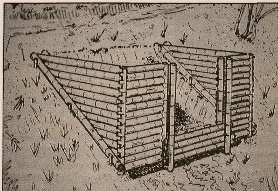
Fosa en tierra complementada con guadua
