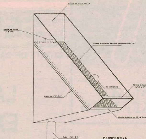
Separador de pulpa tipo Cenicafé construído en lámina
