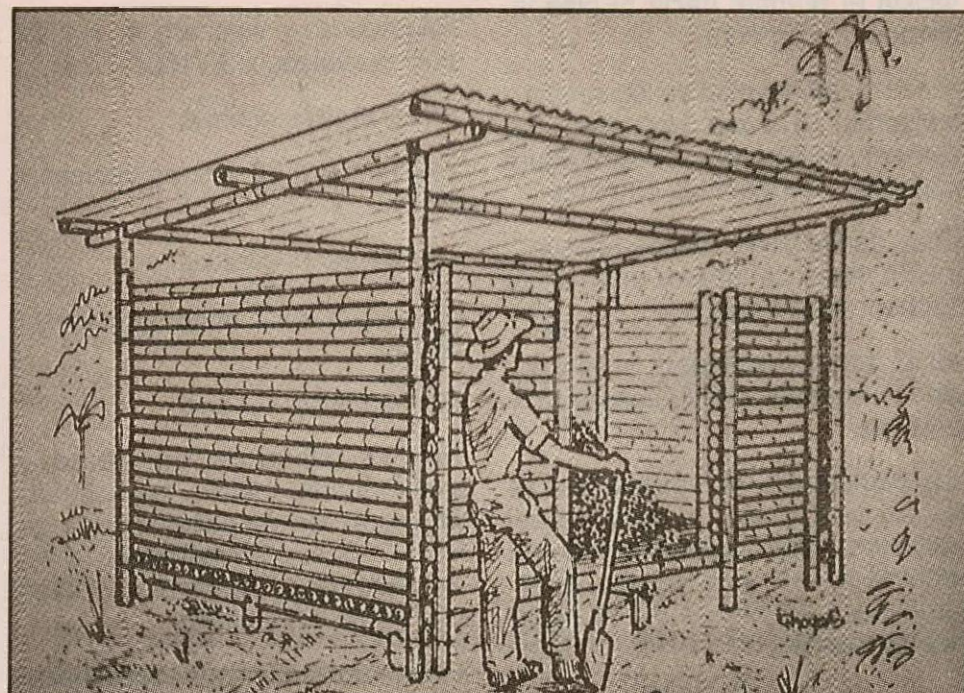
Chiquero de guadua para descomposición de la pulpa. Apropiado para pequeños productores.
